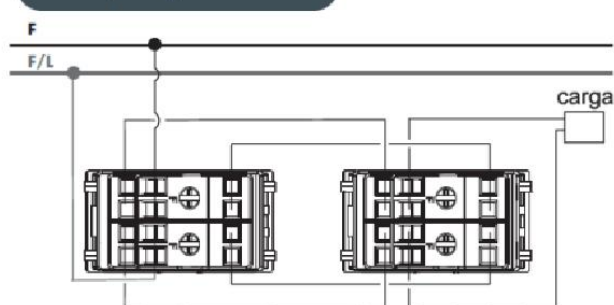
Interruptor Bipolar Paralelo
