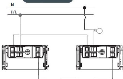
Interruptor Paralelo
