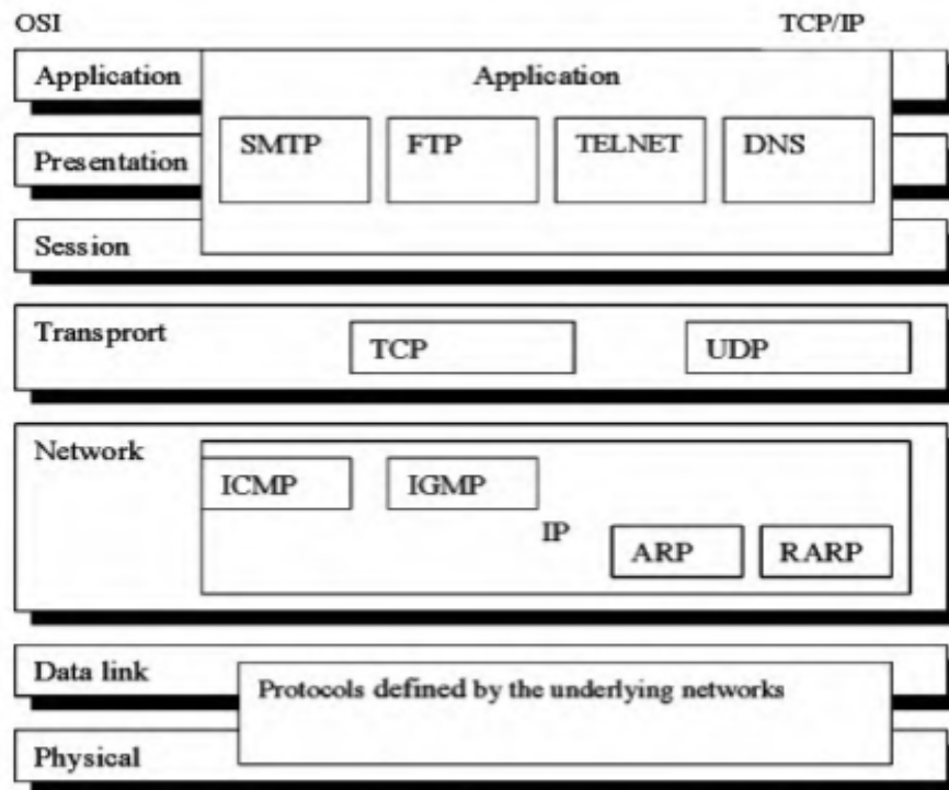
Hình 2.1 Mô hình OSI và mô hình kiến trúc của TCP/IP
