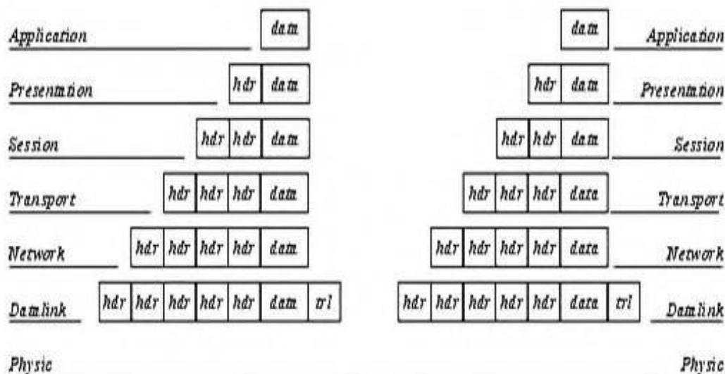
Hình 2.3: Phương thức xác lập các gói tin trong mô hình OSI
