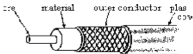
Hình 4.2: Cáp đồng trục
