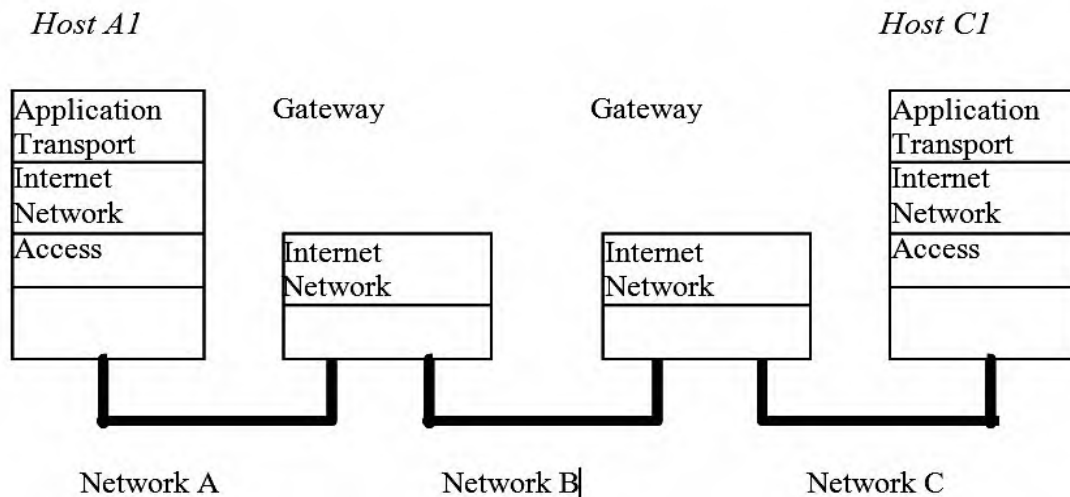
Hình 5.7: Định tuyến giữa hai hệ thống
