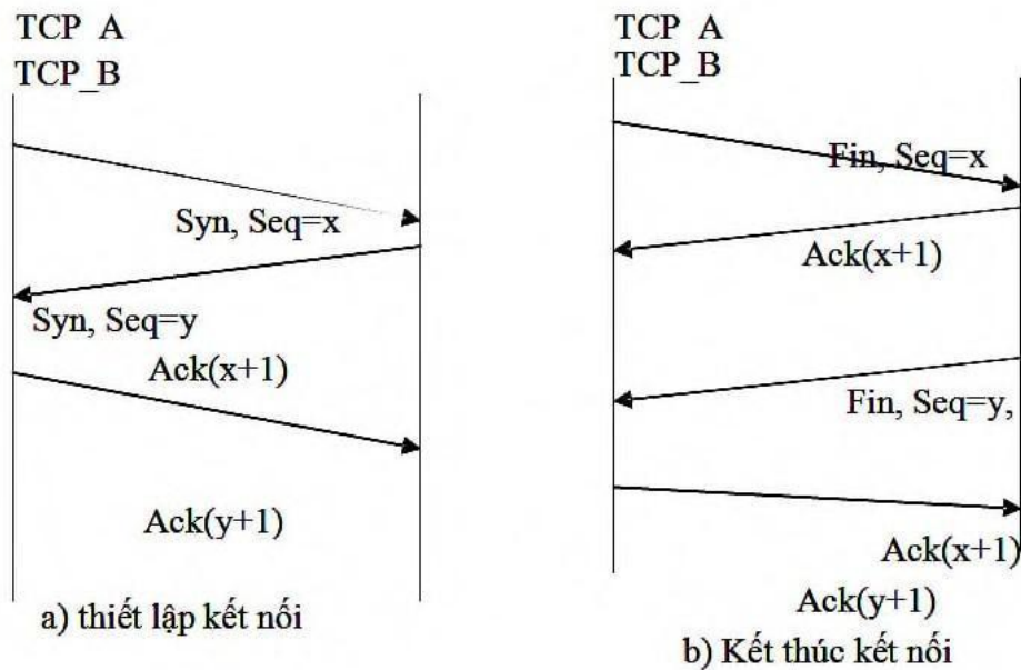
Hình 5.15: Quá trình kết nối theo 3 bước
