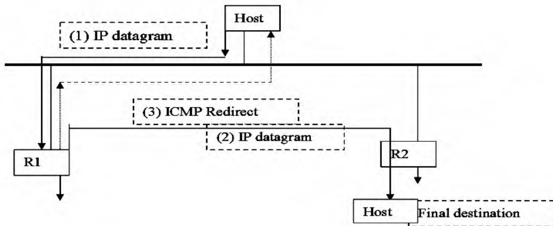
Hình 5.8: Mô tả một ứng dụng của giao thức ICMP thực hiện việc định tuyến lại
