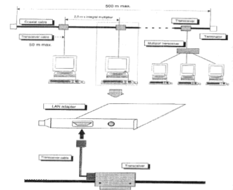
Hình 4.7: Kết nối theo chuẩn 10BASE5
