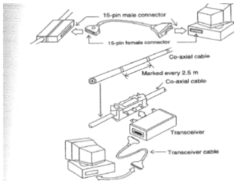
Hình 4.3: Kết nối bằng Transceiver
