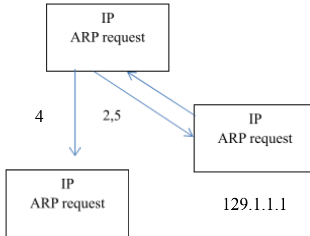
Hình 5.12: Tiến trình ARP
