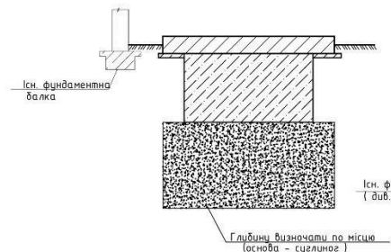
3 - 3 (опалубка)
