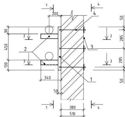
Опора ОП1 ( для цегляних стін)
