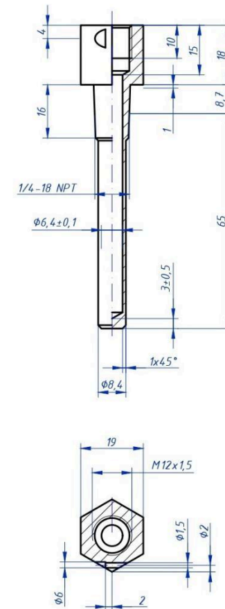
Гільза Delta SE
