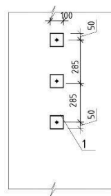
4 - 4
