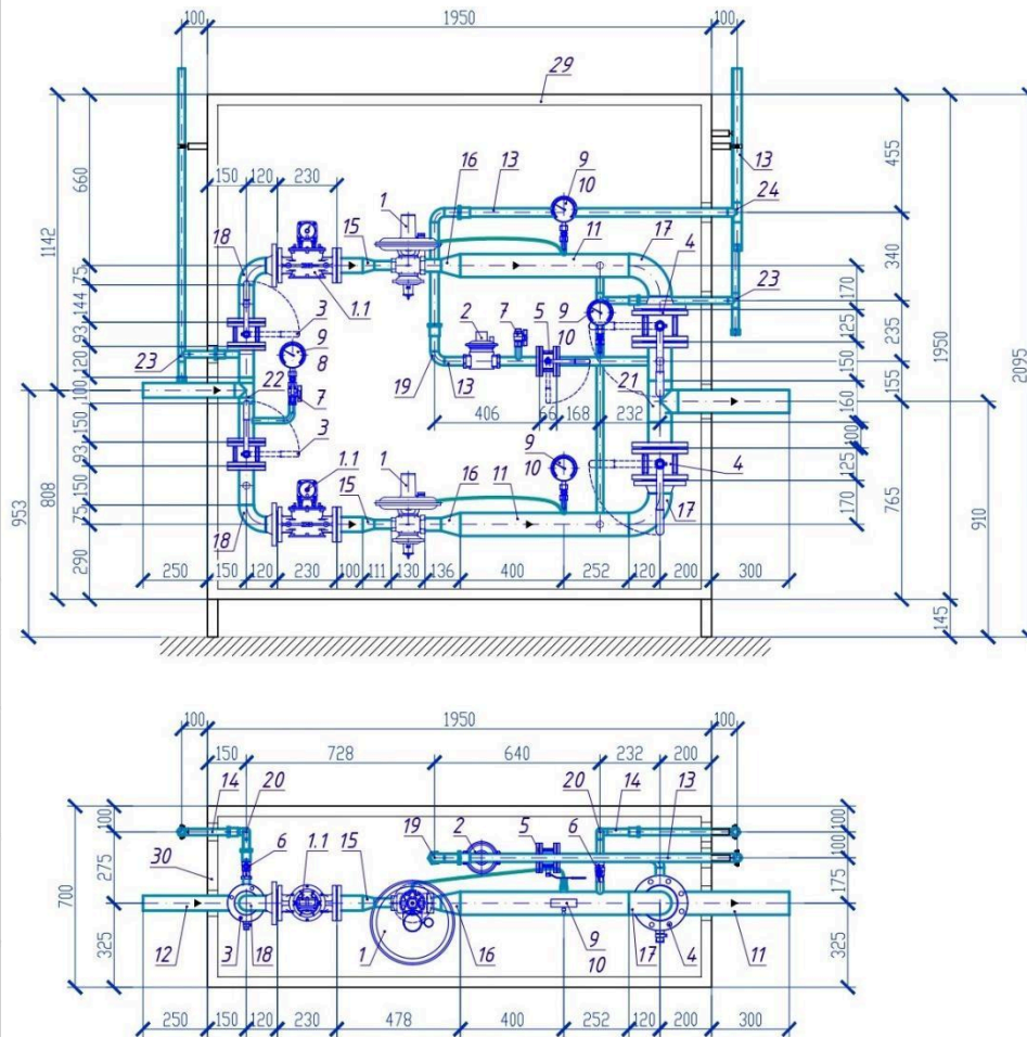
Схема монтажу обладнання ШГРП
