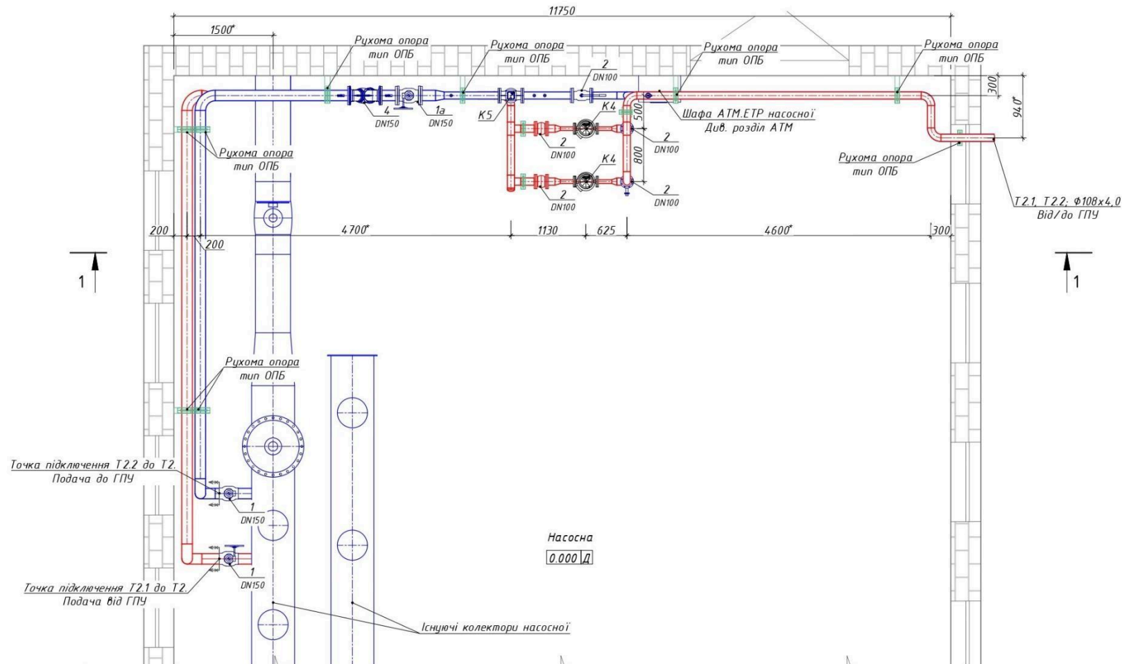
Трасування трубопроводів насосної. План на відмітці 0,000
