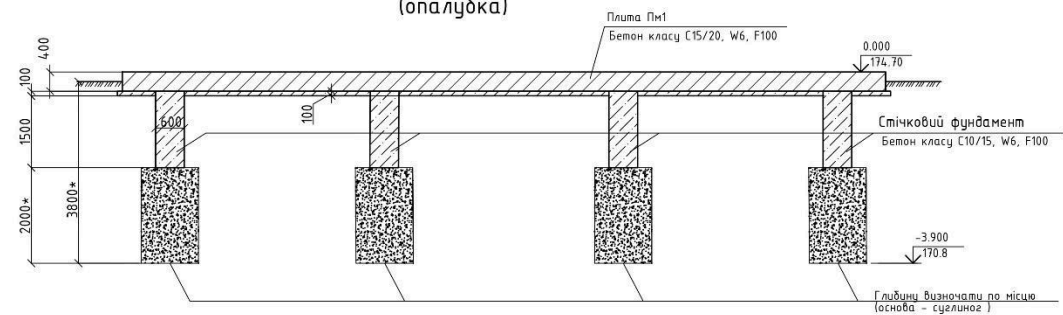
3 - 3 (опалубка)
