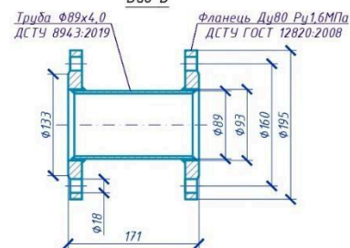
Вид В
