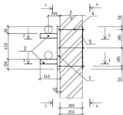
Опора ОП2 ( для стінових панелей)
