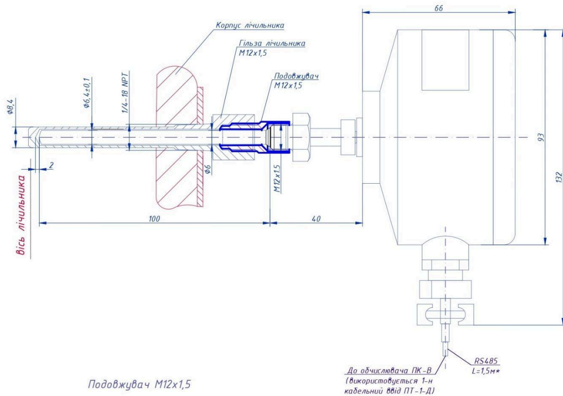
Гільза в лічильнику
