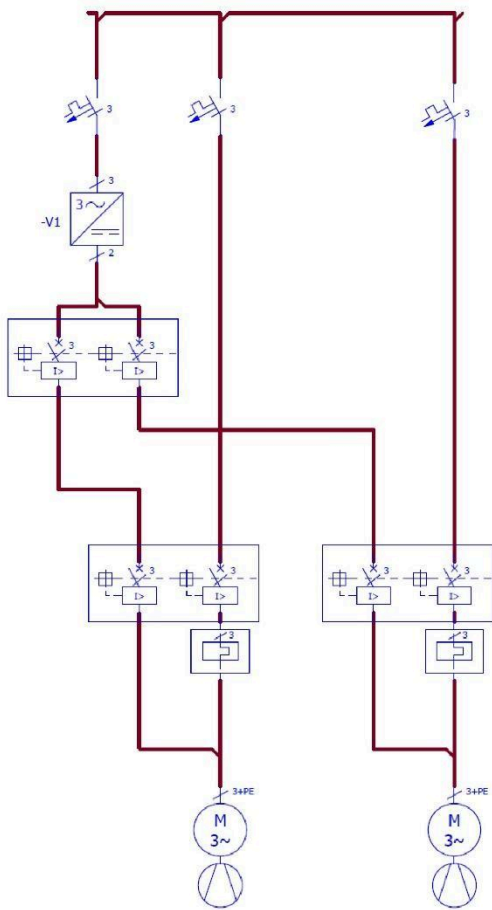
Схема підключення ЧП
