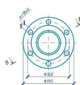
З'ємна котушка під лічильник Ф89х4,0; L=171мм
