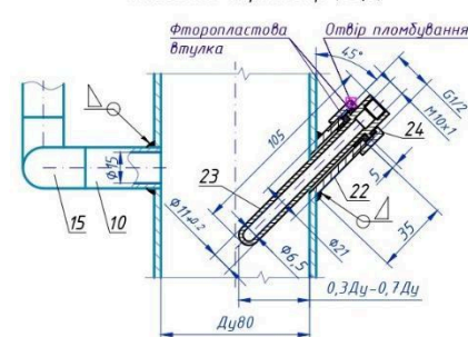
Гільза під термометр (1,2,5)
