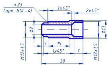
Подовжувач M12x1,5
