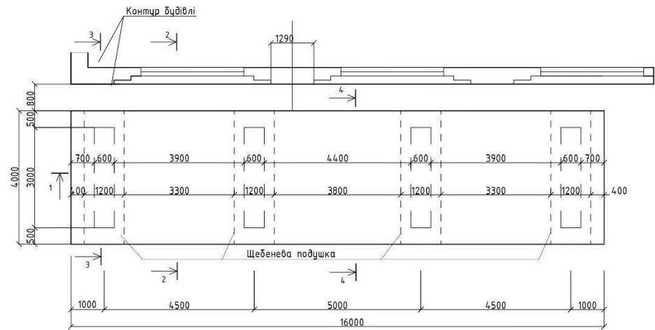
1 - 1 (опалубка)
