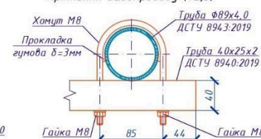
З'ємна котушка під лічильник Ф89х4,0; L=171мм
