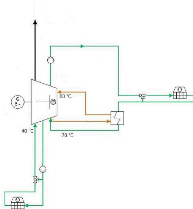
Принципова схема системи охолодження агрегату
