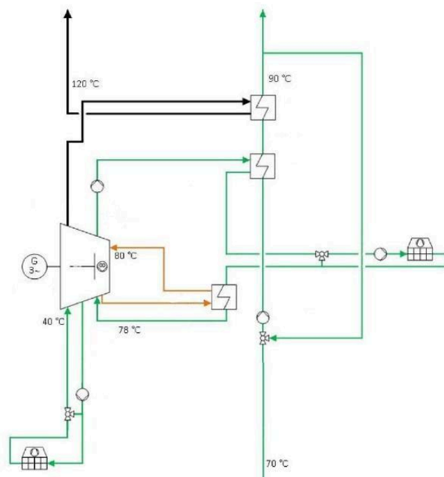
Принципова схема системи роботи когенераційної установки
