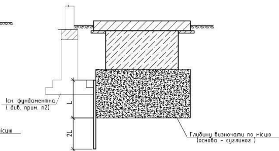
2 - 2 (опалубка)
