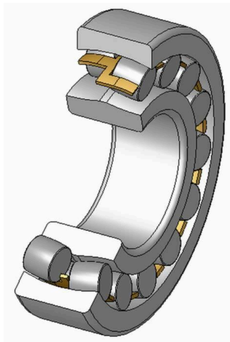
Рис. 2.12. Самоустановлювальний радіальний роликовий підшипник
