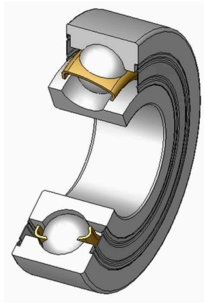
Рис. 2.4. Радіальний підшипник
