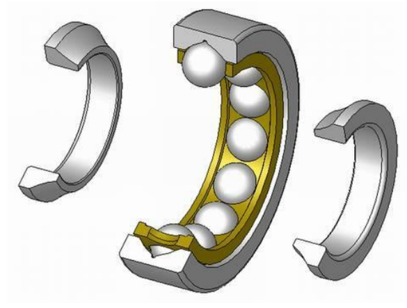
кульковий Рис.2.5. Радіально-упорний кульковий підшипник з чотириточковим контактом
