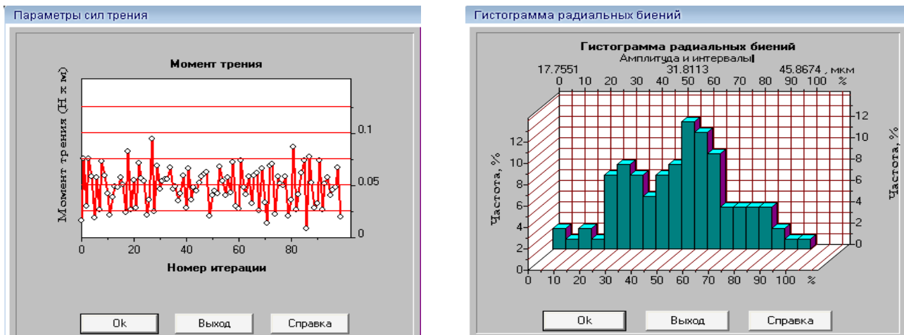
Рис. 3.7. Вікно APM WinBear , для виводу мультиплікації роботи підшипника
