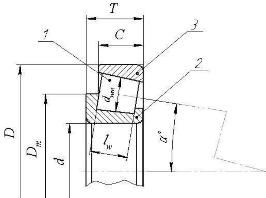
Рис. А3. Ескіз радіально-упорного підшипника з конічними роликами
