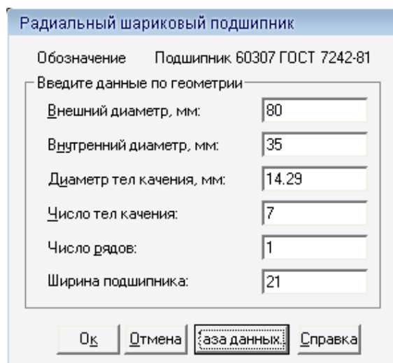
Рис. 3.2. Вікно APM WinBear для завдання геометричних розмірів підшипника
