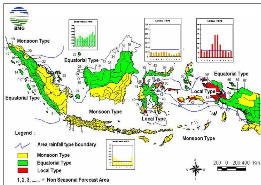
Gambar 2.4 Pola hujan di Indonesia (BMG, 2007)
