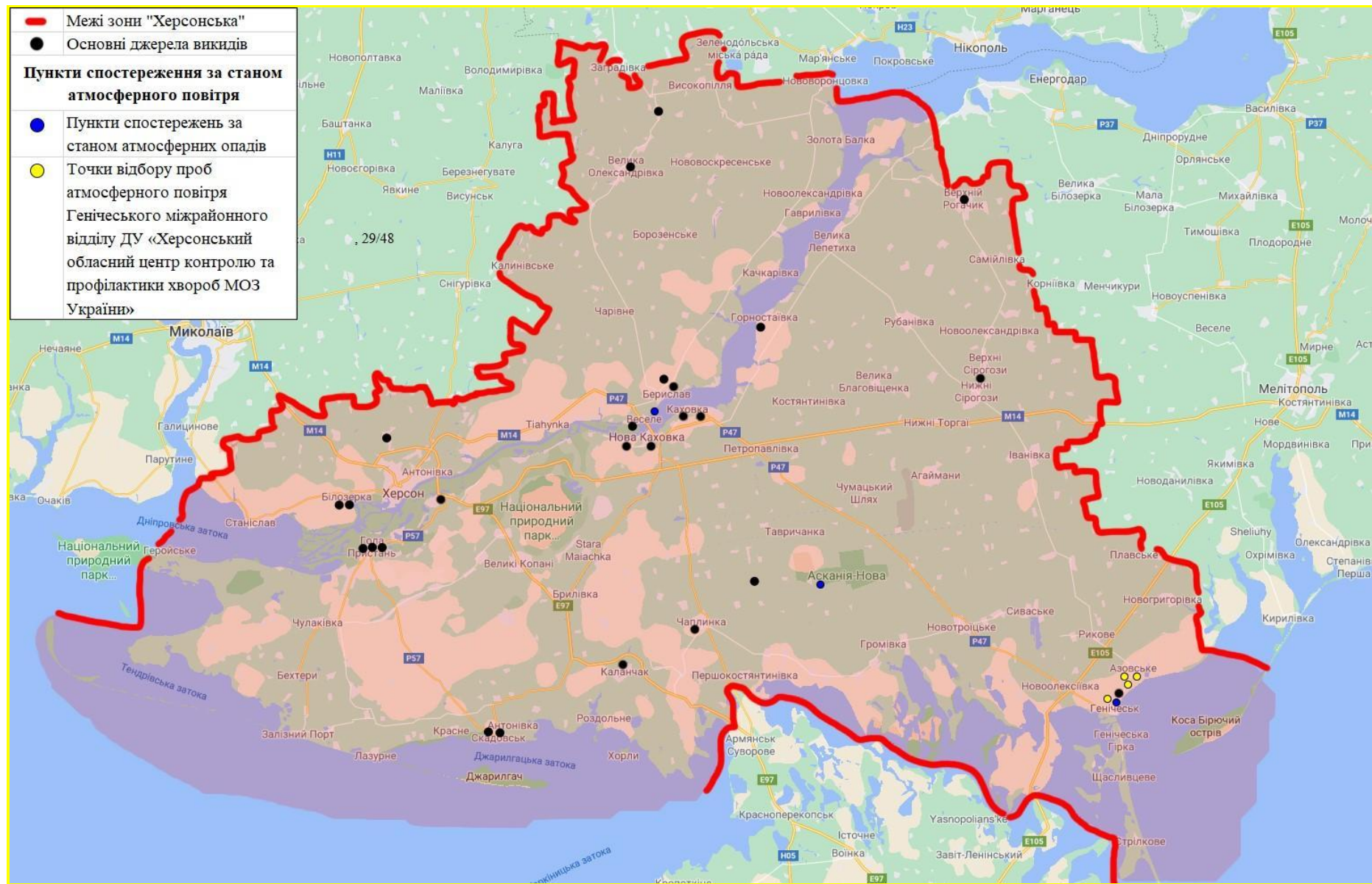
Мал. 3. Карта розташування основних джерел викидів та пунктів спостереження за станом атмосферного повітря зони «Херсонська»
