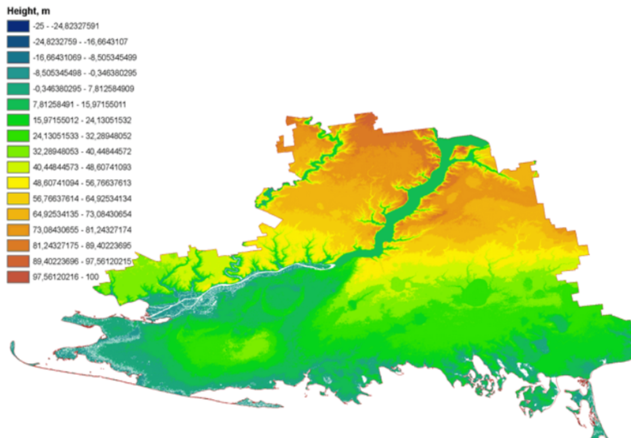
Мал. 2. Рельєф зони «Херсонська»
