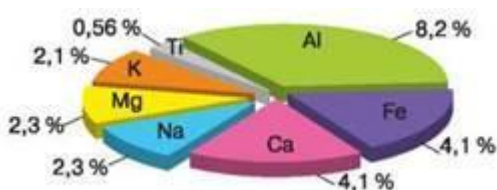
Рис. 44. Діаграма поширення металічних елементів у природі
