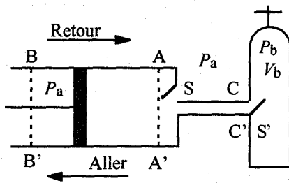
Fig. 2 : Compresseur
