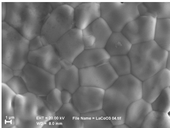
Gambar 1. Foto SEM permukaan membran LaCo 1-x Ni x O 3-δ dengan kalsinasi 1250°C selama 9 jam[Nomor Rujukan]
