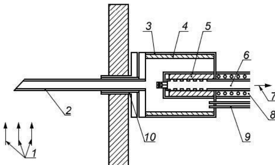
1 - поток отходящего газа; 2 - зонд; 3 - водонепроницаемый кожух; 4 - нагреватель; 5 - фильтр; 6 - трубка для отбора проб; 7 - газ; 8 - нагреватель; 9 - трубка для подачи калибровочного газа; 10 - штуцер для подсоединения зонда
