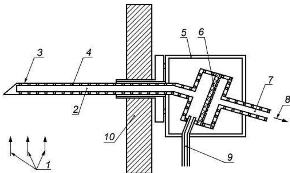
Рисунок 6 - Пример компоновки системы экстрактивного отбора проб с блоком электронагрева зонда и защитной трубкой для зонда
