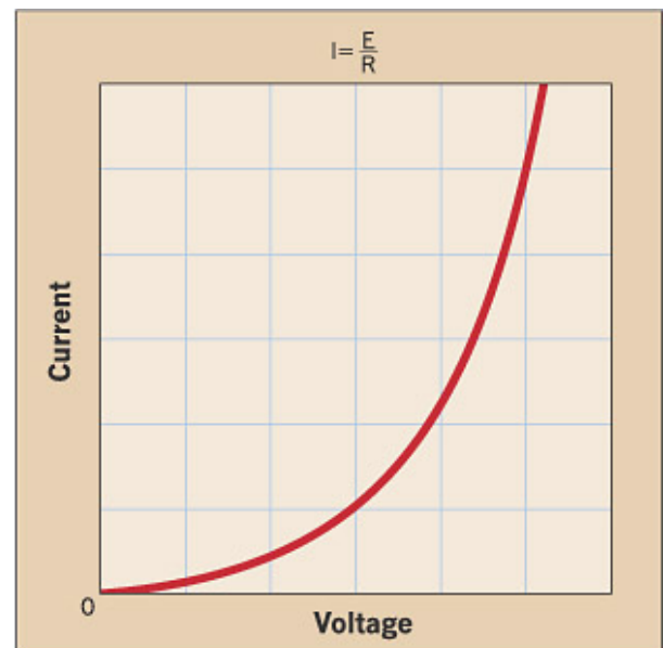
Figure 11.1 B: Non Linear Load
