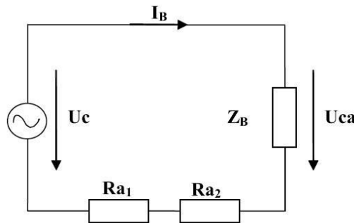
Figura 2. Esquema del circuito de contacto
