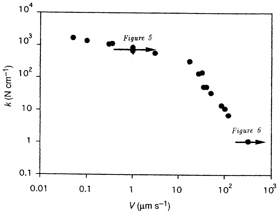
Figure 4 - Transition entre le régime permanent et le régime fixe-glisse. Représentation logarithmique en fonction des variables (V, k) , avec un palet de masse m = 1, 2 kg. Chaque point correspond à une expérience où l'on observe la disparition du régime fixe-glisse. Les flèches indiquent les régions étudiées plus en détail dans les figures 5 et 6.
