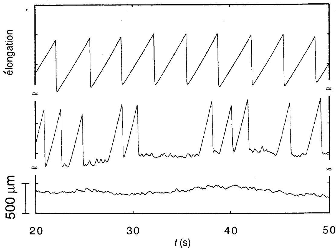
Figure 6 - Transition, lorsque k = 1 \text{ N. cm}^{-1} et m = 1, 2 \text{ kg} , - voir flèche sur la figure 4. Les enregistrements de l'élongation du ressort ont été décalés les uns au-dessus des autres pour être lisibles. De haut en bas, les trois vitesses de tirage sont respectivement : 275; 525; et 890 \text{ } \mu\text{m.s}^{-1}
