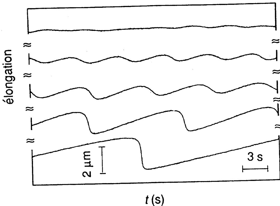
Figure 5 - Transition, lorsque k = 740 \text{ N.cm}^{-1} et m = 1, 2 \text{ kg} ; voir flèche sur la figure 4. Les enregistrements de l'élongation du ressort ont été décalés les uns au-dessus des autres pour être lisibles. De bas en haut, les cinq vitesses de tirage sont respectivement : 0,25 ; 0,42 ; 0,59 ; 0,75 et 1 \mu\text{m.s}^{-1} .
