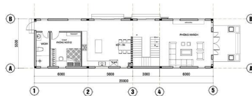
MẶT BẰNG TẦNG TRỆT TL1/100
