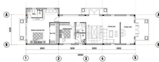
MẶT BẰNG LẦU 01 TL1/100
