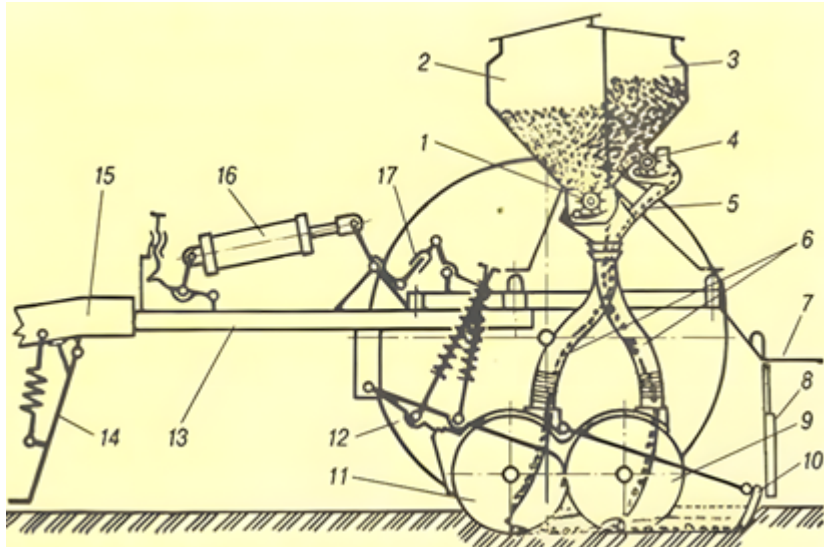
Рис. 3.1.1. Схема робочого процесу зернотукової рядкової сівалки СЗ-3,6А:
