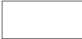
Gambar 1. Gambar Segiempat
