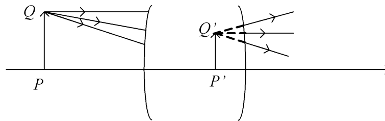
Système centré
