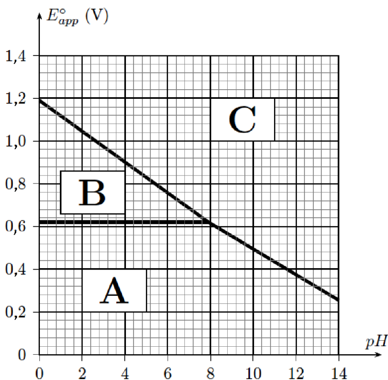
Figure 5: Diagramme potentiel standard apparent de l'iode en fonction du pH.
