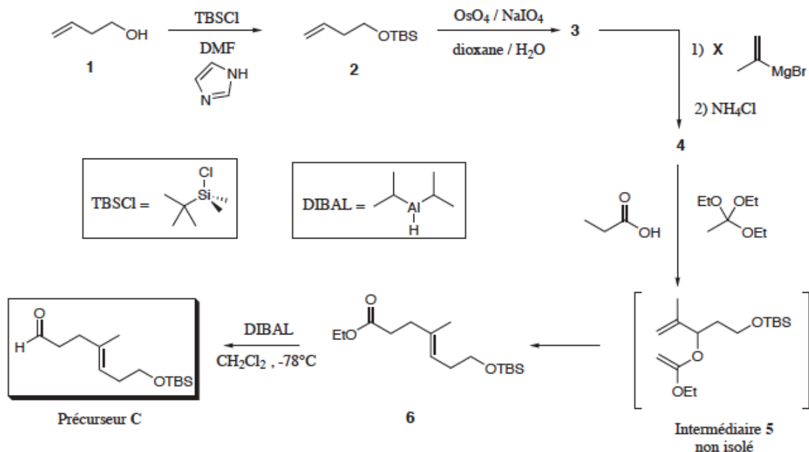
Figure 7: Préparation de l'aldéhyde C.
