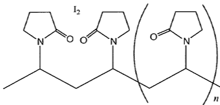
Figure 4: Représentation simplifiée de la PVP-I. Entre parenthèses, on retrouve une entité monomérique de masse molaire égale à 111 g/mol.
