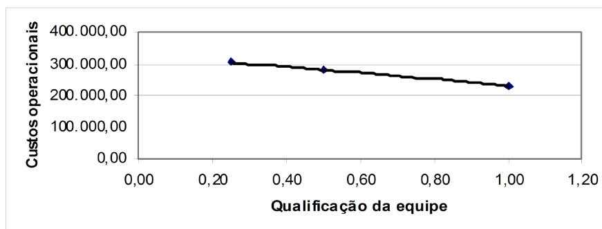
Gráfico 1 - Custos operacionais
