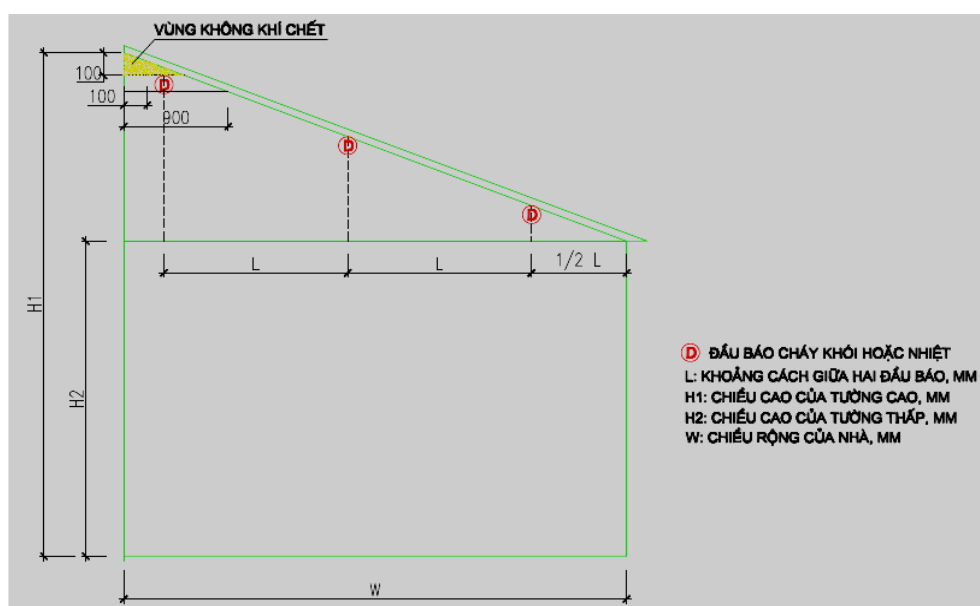
Hình 1: Phương pháp xác định vị trí lắp đặt các đầu báo cháy trên nhà mái dốc
