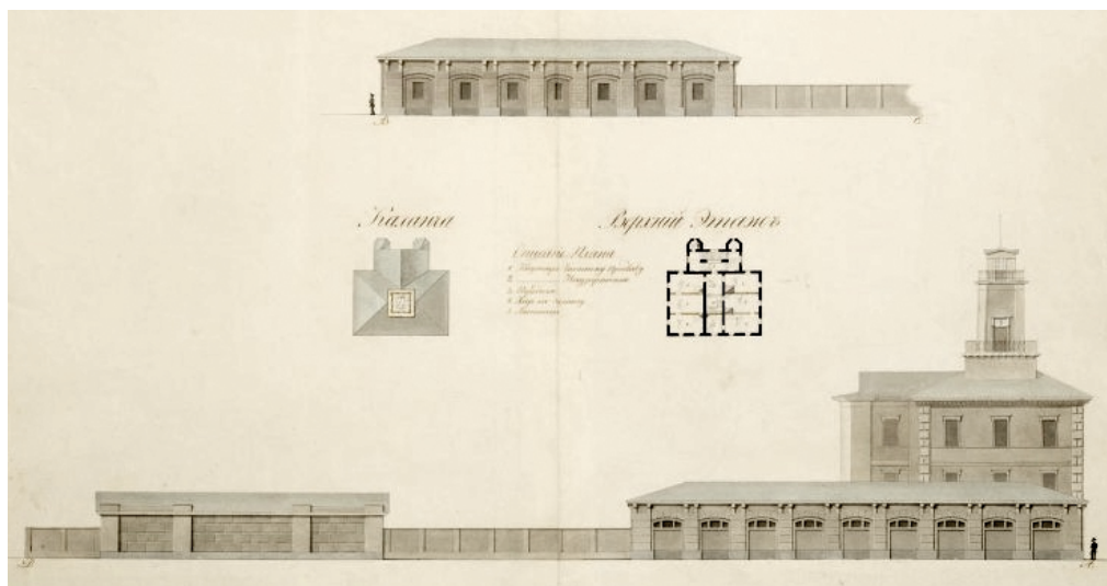
Гильдебрандт А. П. Чертеж «Фасады для постройки служб полиции в 3-ей части г. Царского Села». 1836. ГМЗ "Царское Село"
