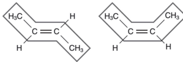
cis-2-butene
