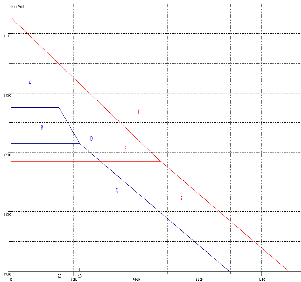
Figure I. Diagrammes E-pH simplifiés du mercure et de l'iode
