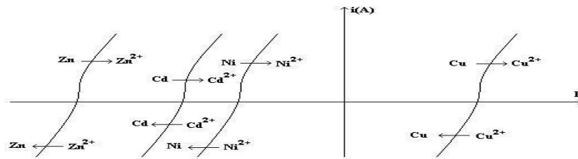
Figure 5 : courbes intensité-potentiel pour différents métaux
