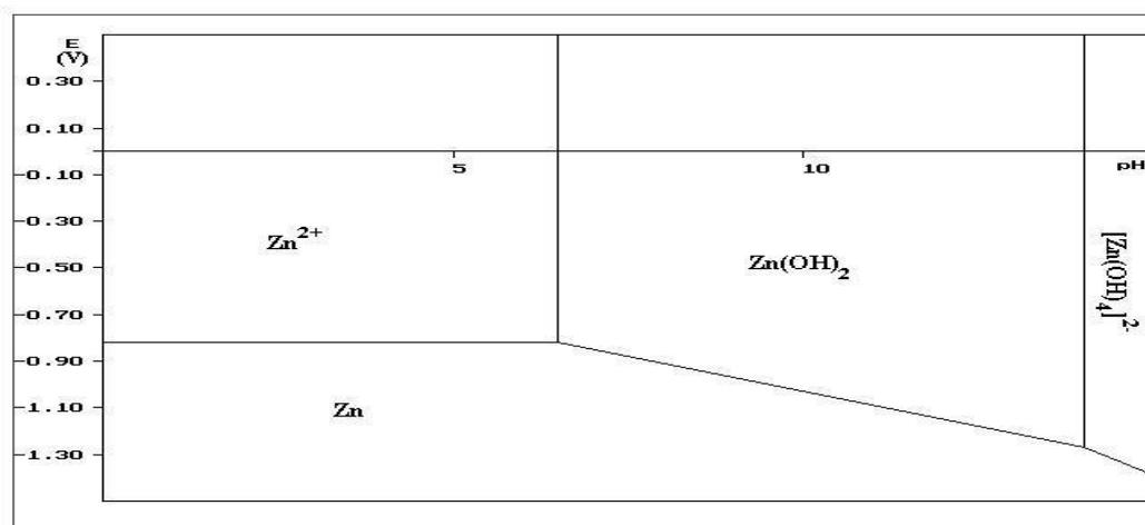
Figure 2 : diagramme potentiel-pH du zinc
