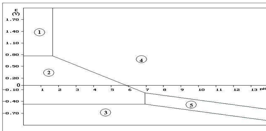
Figure 3 : diagramme potentiel-pH simplifié du fer
