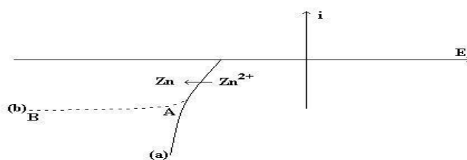
Figure 4 : courbes intensité-potentiel du zinc a) Zn^{2+} concentré b) Zn^{2+} dilué
