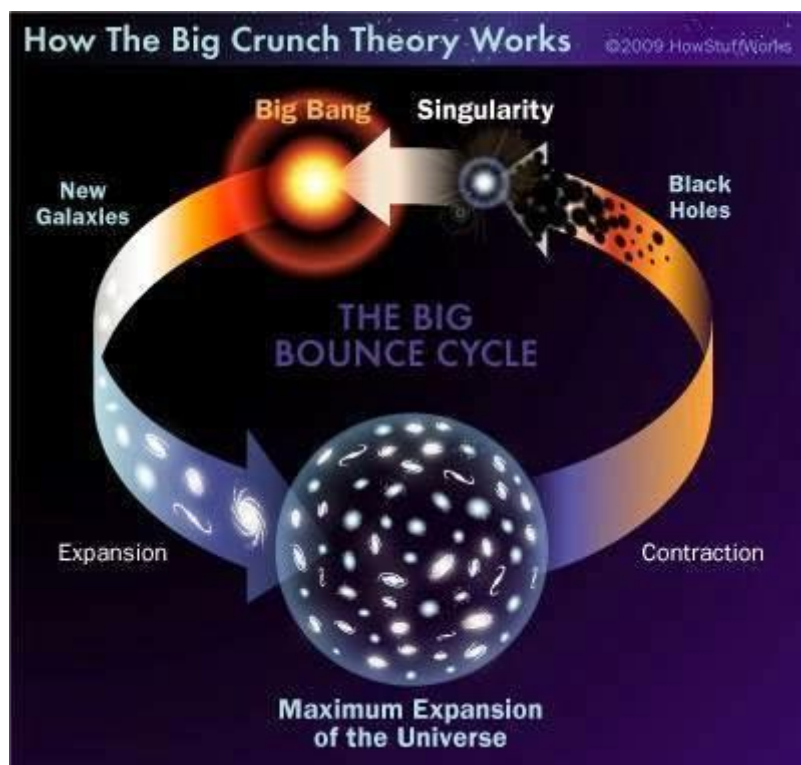
Ilustração de dois instantes da Singularidade descrita por Stephen Hawking, no Big-Bang e no Big Crunch ou, respectivamente no início e no fim desse Universo – Imagem da Internet.
