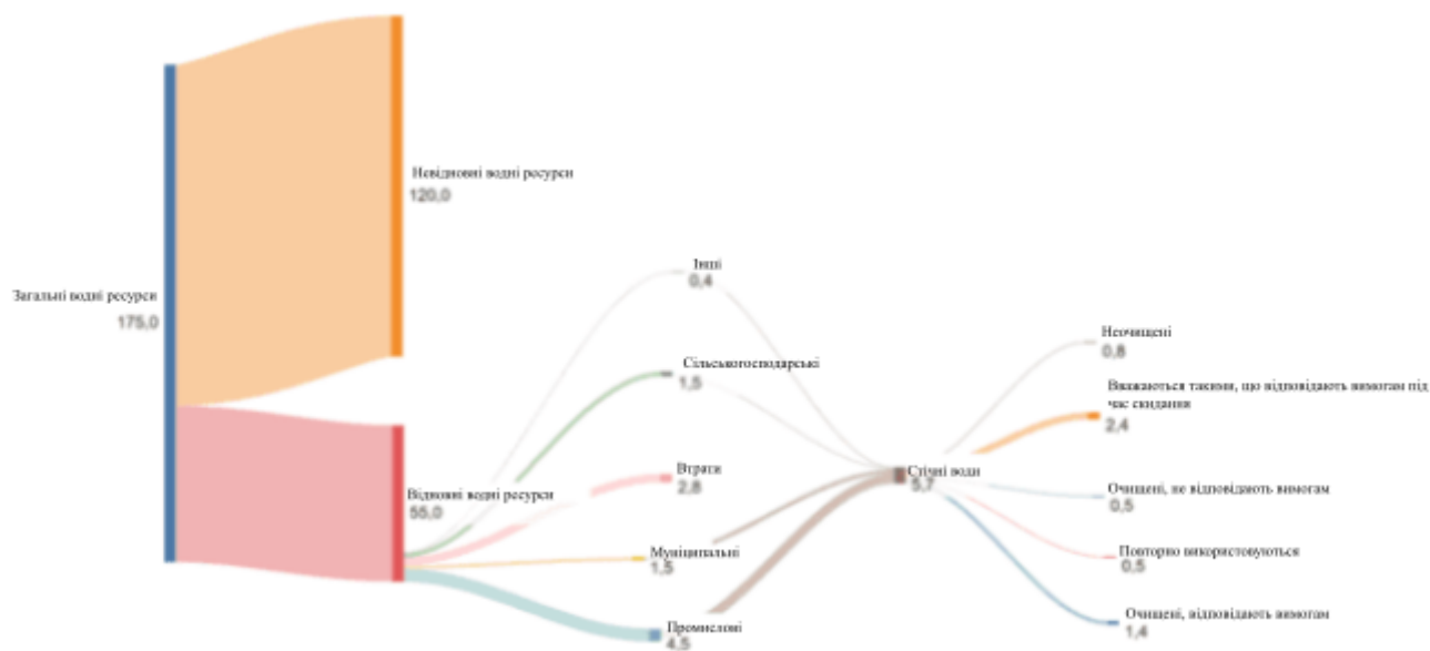
Рисунок А1. Розподіл водних ресурсів в Україні в км 3 /рік. За оцінками /9/, /10/ і Wise Europa
