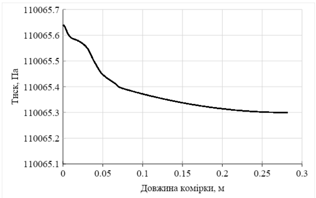
Рис. 2. Результати імітаційного моделювання процесу формоутворення комірки захисної надувної упаковки зі зворотним клапаном, який має чотири вихідних повітряних потоки:
