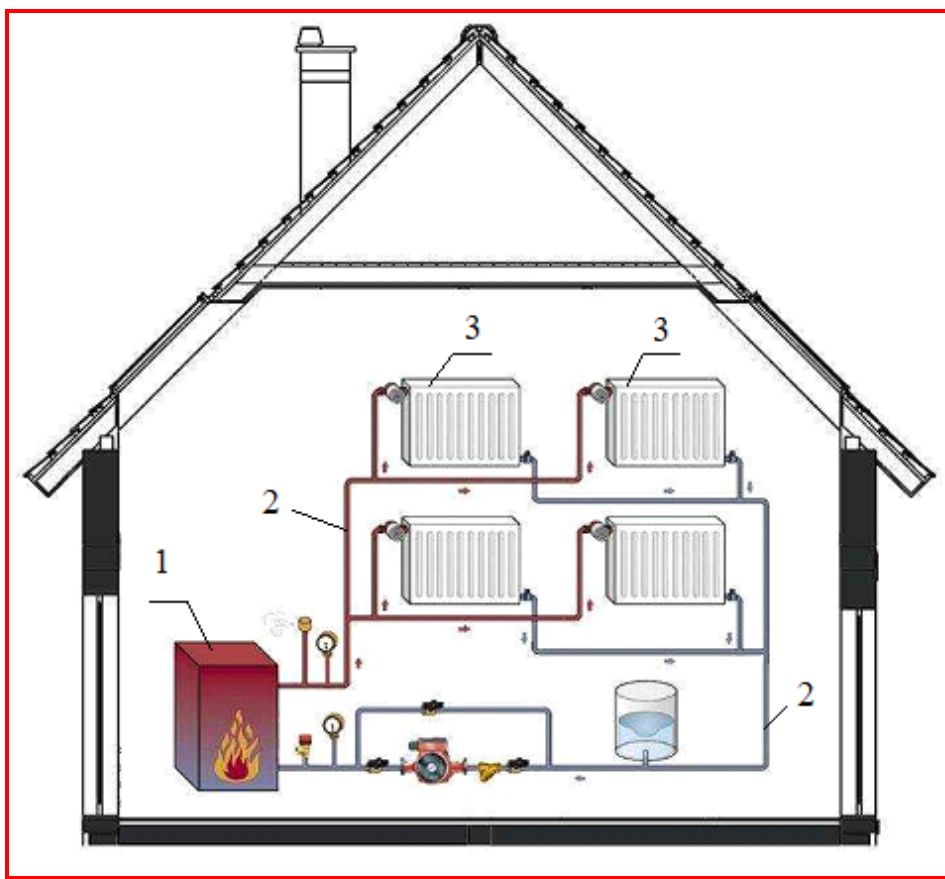
Рисунок 4. – Система отопления: 1 – источник теплоты (котел); 2 – теплопроводы; 3 – отопительные приборы (радиаторы)
