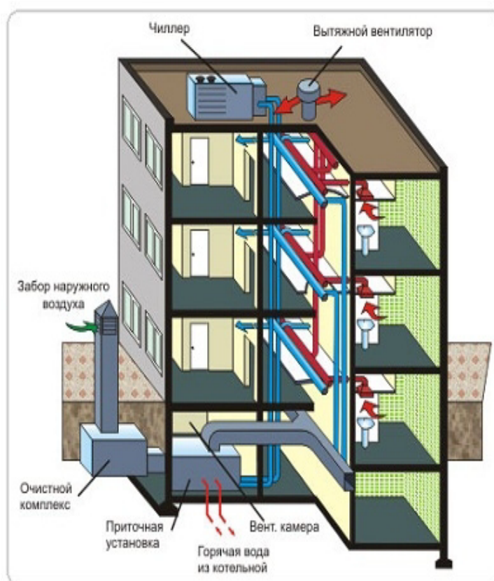
Рисунок 6. – Кондиционирование воздуха
