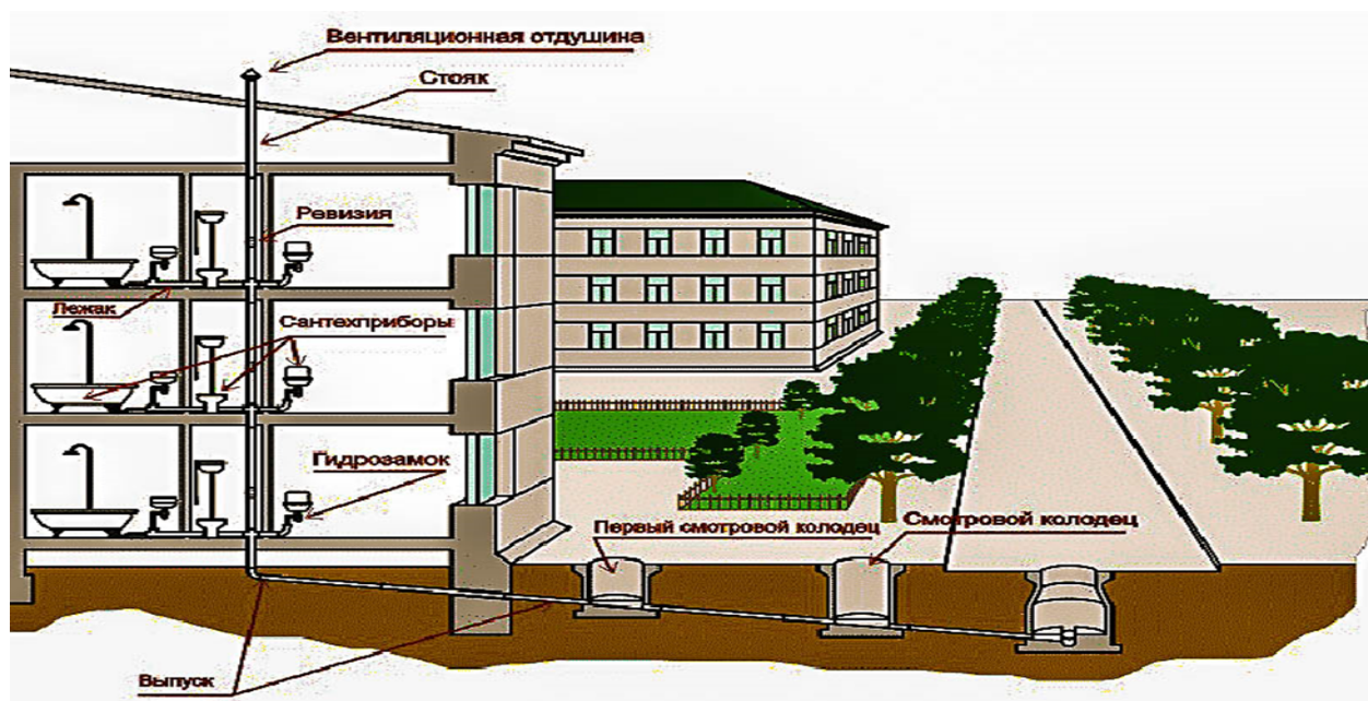
Рисунок 2. – Канализация здания
