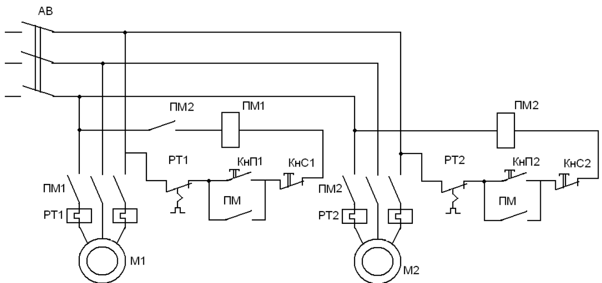
Схема реверсивного пуска асинхронного электродвигуна з коротко замкненим ротором, з блокуванням на магнітному пускачу.
