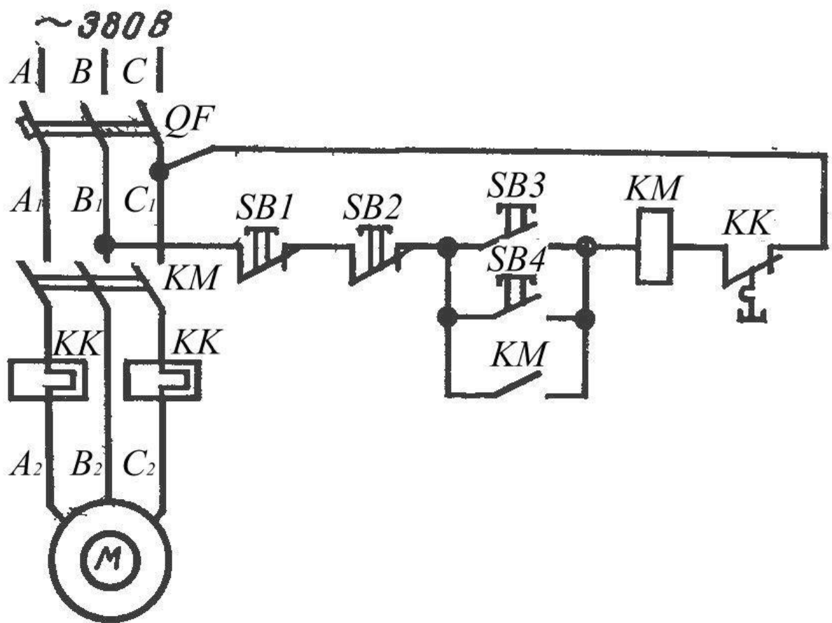
Схема пуску асинхронного електродвигуна з двох робочих місць.
