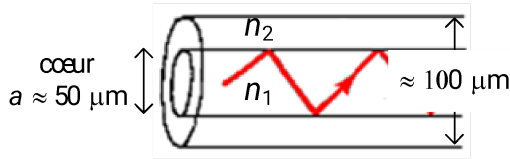
Fig. 1 - Guide d'ondes diélectrique
