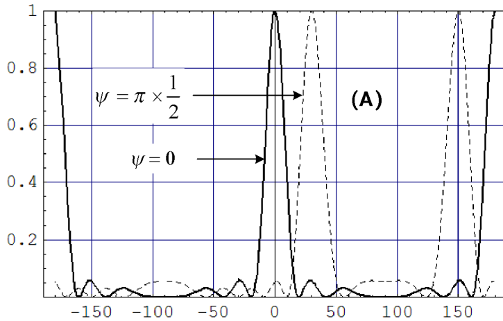
Fig. 13 – Quelques résultats relatifs à un réseau de six antennes espacées de
