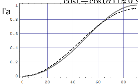
Fig. 11 - La fonction \cos[\pi \cos(\theta)/2] en trait plein et son approximation en pointillés. L'abscisse est en degrés.
