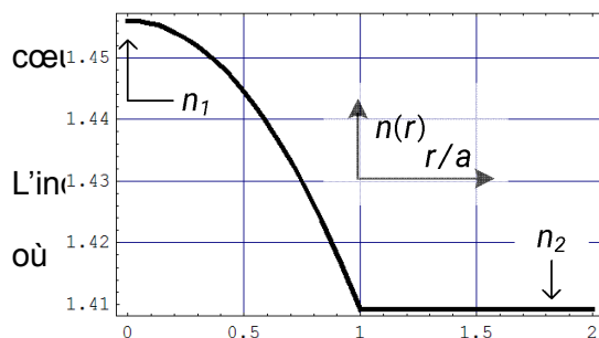
Fig. 5 - Un profil d'indice, F(u) = u^2 .
