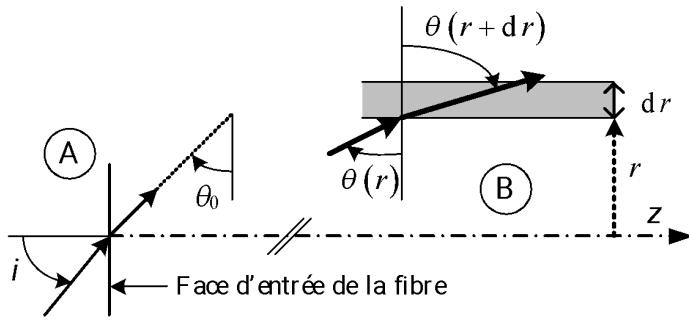
Fig. 6 – En A, représentation de l'angle externe d'entrée dans la fibre i , et de l'angle interne \theta_0 ; en B, représentation de la loi de Descartes dans un plan méridien et pour deux dioptries plans situés en r et en r + dr .
