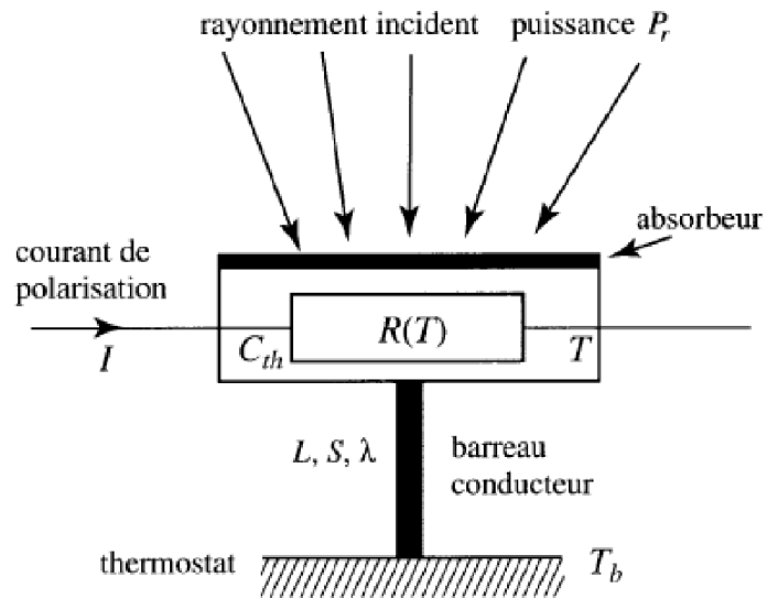
Figure 1 - Schéma d'un bolomètre
