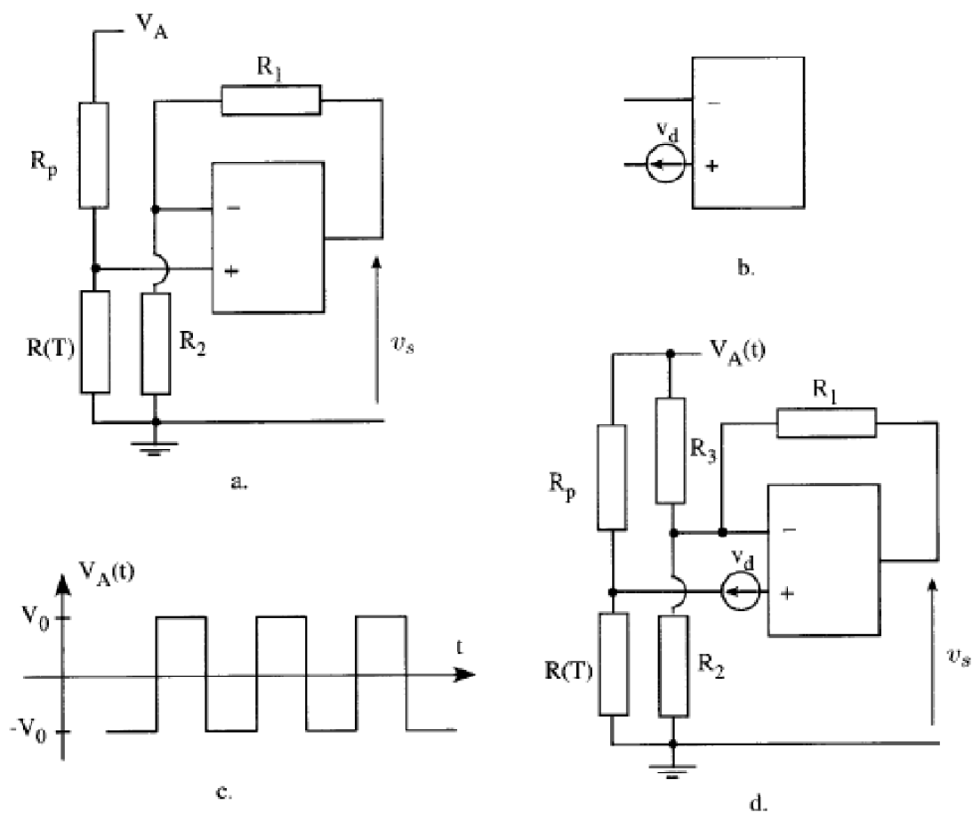
Figure 3 - Électronique de lecture du bolomètre
