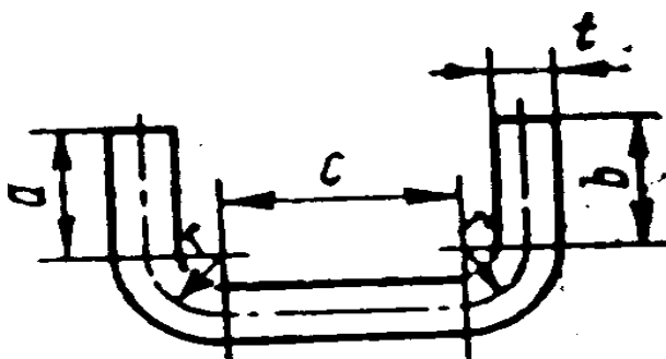
Рис. 5. Определение длины заготовок.
