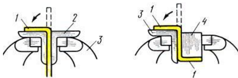
Рис. 97. Гибка двойного угольника: 1 - заготовка, 2 - нагубники, 3 - тиски, 4 - брусок-подкладка
