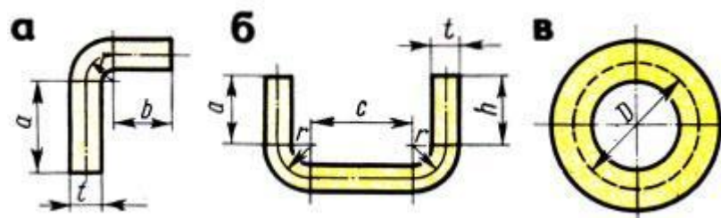
Рис. 94. Схемы для определения длины заготовок: а - угольника с внутренним закруглением, б - скобы с закруглением, в - кольца
