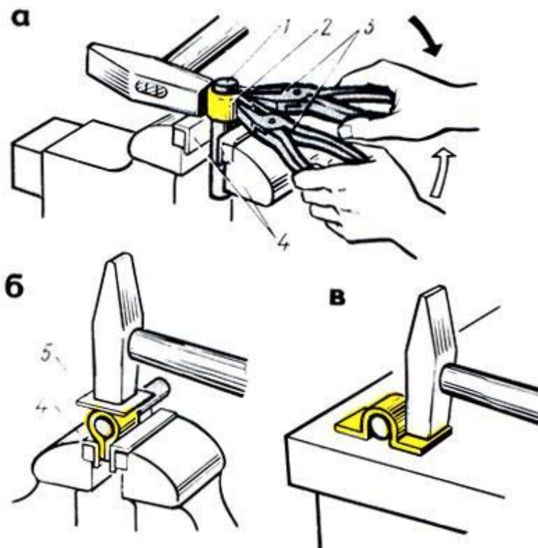
Рис. 98. Гибка хомутика: а - изгибание плоскогубцами на оправке, б, в - формирование хомутика; 1 - оправка, 2 - хомутик, 3 - плоскогубцы, 4 - нагубники, 5 - мягкая прокладка
