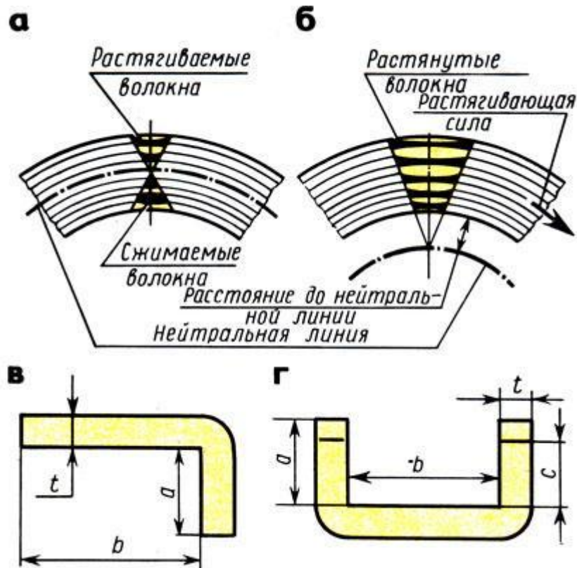
Рис. 93. Напряжения в заготовке при простом изгибе (а), при изгибе с растяжением (б), схемы для определения длины заготовок (в, г)
