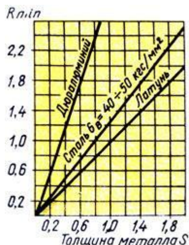
Рис. 95. График для определения радиуса загиба листового и полосового материала
