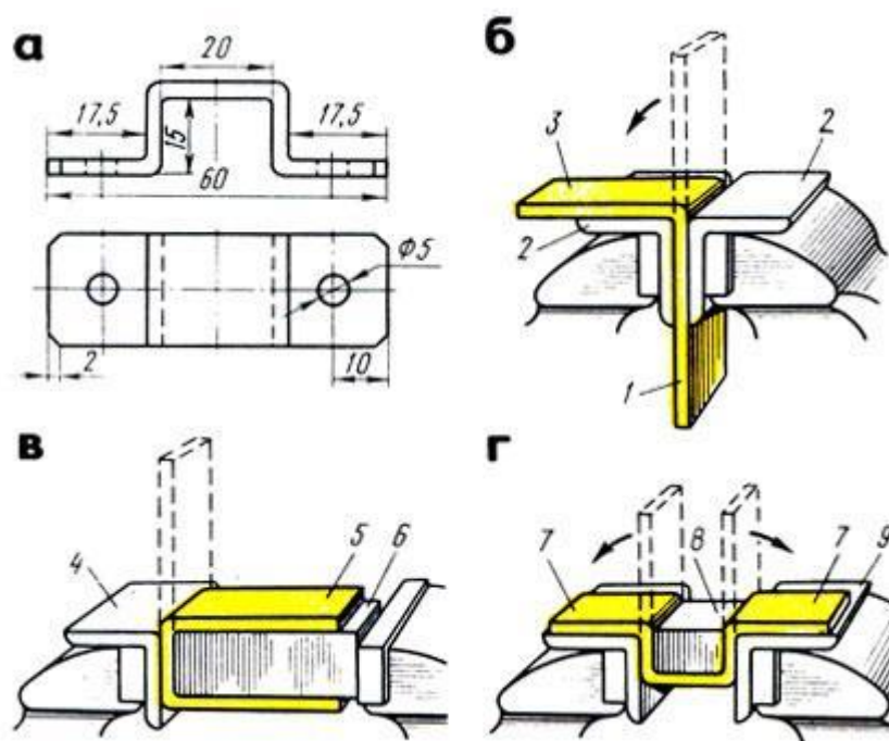
Рис. 96. Гибка прямоугольной скобы: а - схема для определения длины скобы, б - гибка одного конца, в - гибка второго конца, г - формирование скобы, 1 - заготовка, 2 - нагубники, 3, 5 - концы скобы, 4, 9 - угольники, 6 - большой брусок (оправка), 7 - лапки, 8 - меньший брусок (оправка)
