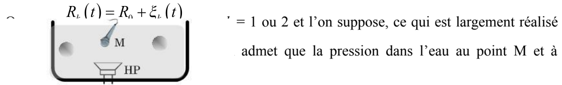
Fig. 2 - Deux bulles d'air dans l'eau, excitées par le haut-parleur HP. L'hydrophone M détecte le signal acoustique produit par les oscillations forcées des bulles.
