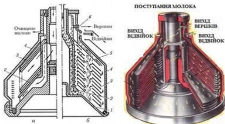
Рис. 9.7. Принципові схеми роботи сепараторів молокоочисника (а) і віддільника вершків (б) 1 – корпус барабана; 2 – тарілотримач; 3 – пакет тарілок; 4 – накривка барабана; 5 – верхня роздільна тарілка; 6 – канал виходу вершків
