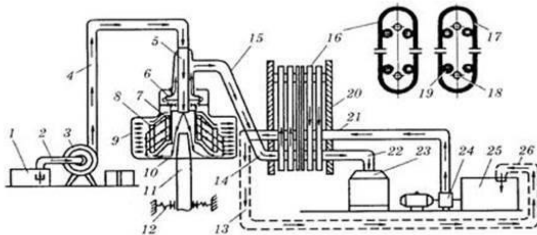
Рис. 9.2. Конструктивно-функціональна схема очисника-охолодника молока ОМ-1А:
