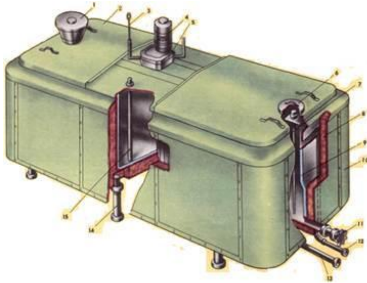
Рис. 9.3. Танк-охолодник молока ТО-2А:
