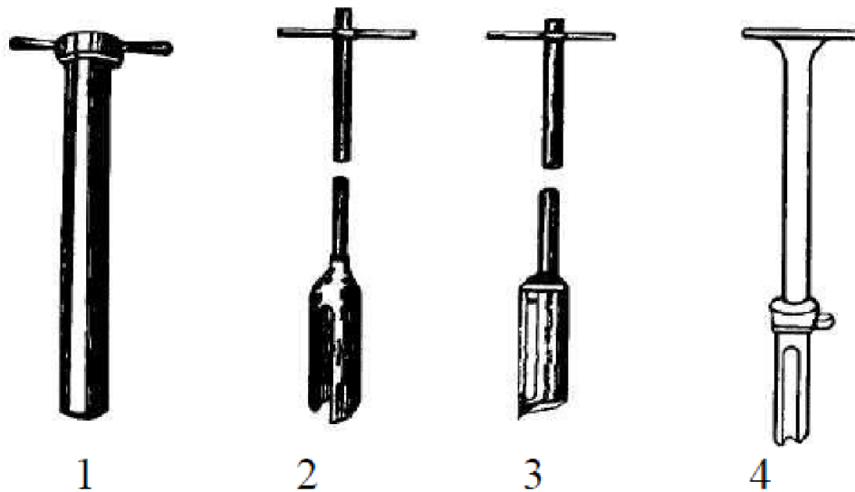
Рис. 2. Бури для відбору проб ґрунту 1. Качинського; 2. Ізмаїльського; 3 – Некрасова, 4 – БН25-15
