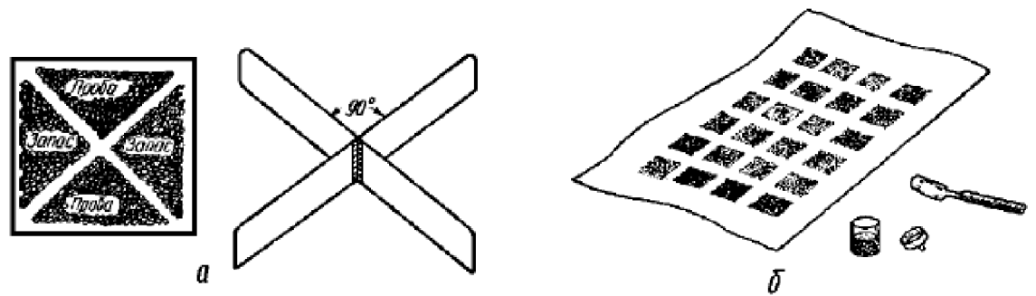
Рис. 5. Відбирання лабораторної та аналітичної проб ґрунтового матеріалу квадратуванням (а) та діленням на квадрати (б)
