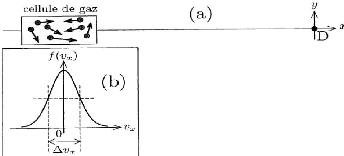
Figure 4: Modélisation de la radiation émise par une assemblée d'atomes ayant une agitation thermique.
