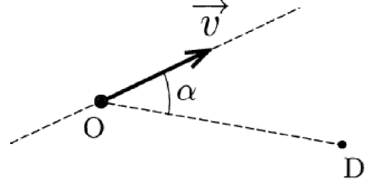
Figure 3: Géométrie relative à la modélisation de l'effet Doppler.
