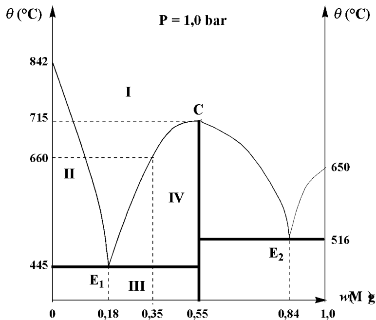
Figure 1 - Diagramme de phases isobare solide-liquide du calcium-magnésium ( P = 1,0 \text{ bar} )
