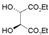
(-)-diéthyltartrate
