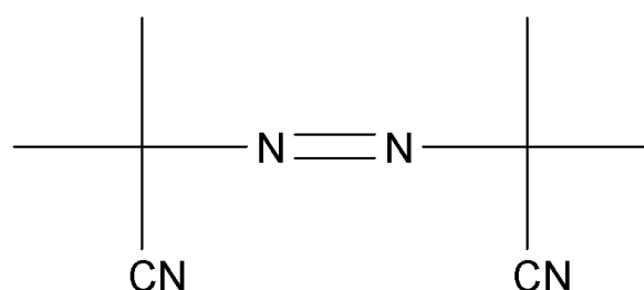
AIBN
