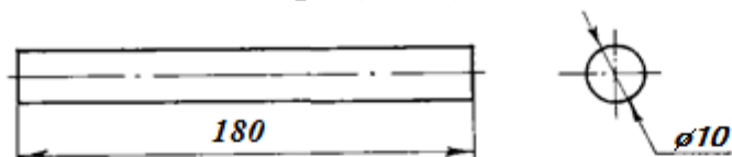
Деталь №7 Опора (1 шт.)
