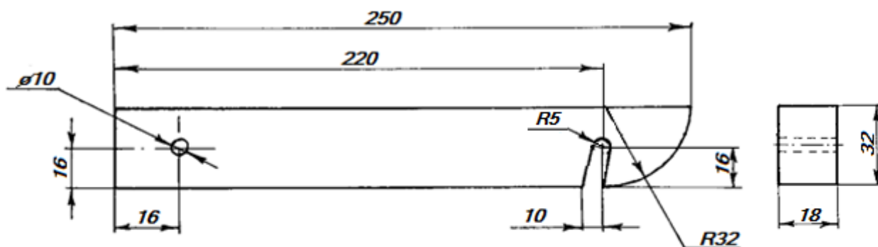
Деталь №2 Опора верхних планок(2 шт.)
