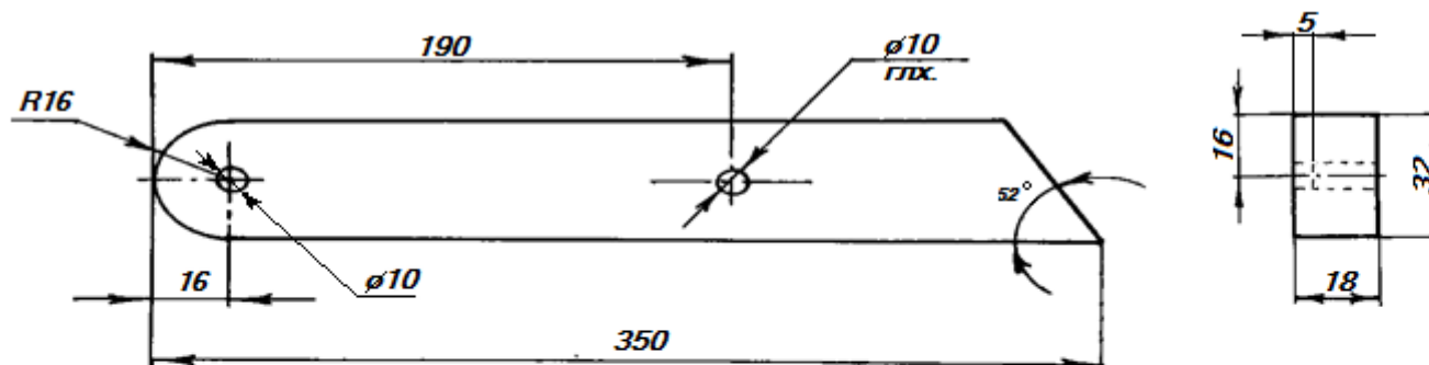
Деталь №5 Ножка(1шт.)
