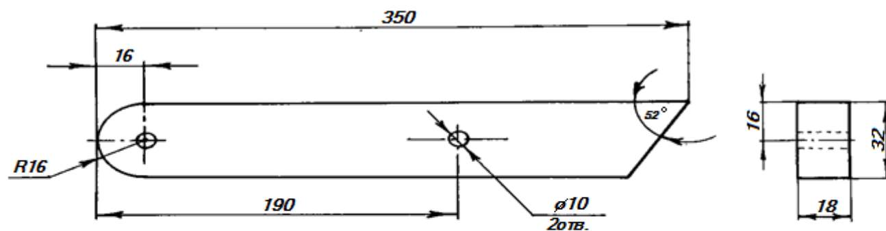
Деталь №4 Ножка(1шт.)
