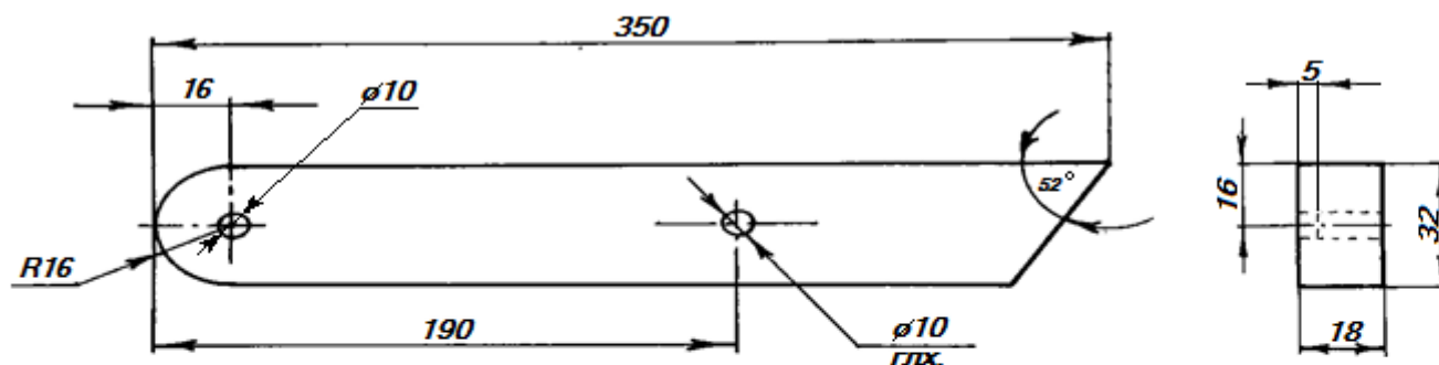
Деталь №4 Ножка(1шт.)
