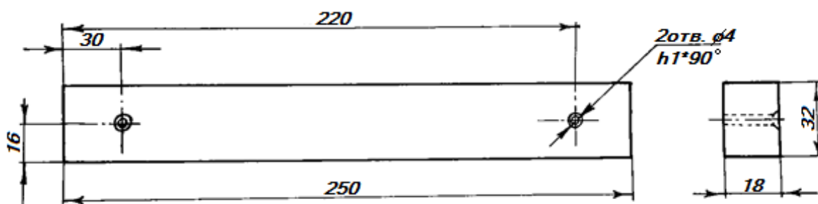
Деталь №2 Опора верхних планок(2 шт.)
