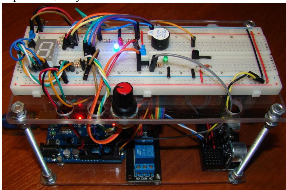
Рисунок 1 – Лабораторний стенд у зборі
