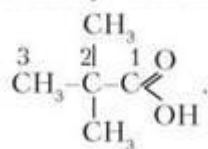
2,2-диметилпропанова кислота
