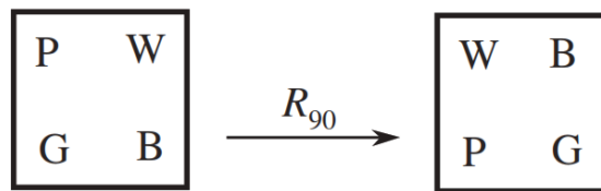
Gambar 1. Persegi PWBG jika Dirotasi 90° Sumber: Gallian (2017)
