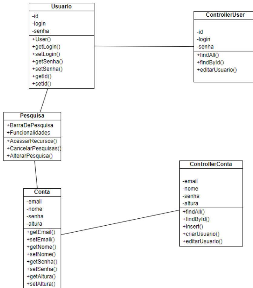
Diagrama de Classes
