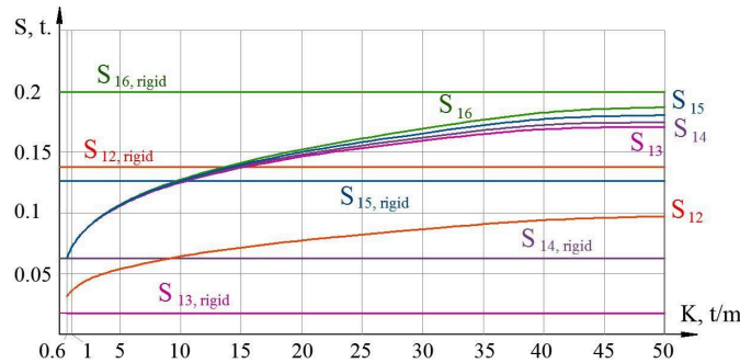
Фиг. 3. Връзка между сеизмичните сили (първият режим на вибрация) ( S_{1i} ) и твърдостта на амортизиращия лагер ( K )
