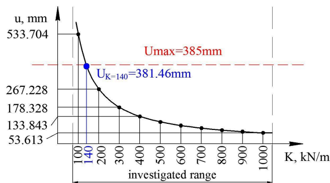
Фиг. 4. Връзка между твърдостта на амортизиращия лагер ( K ) и хоризонталното изместване на долната точка на сградата ( u )
