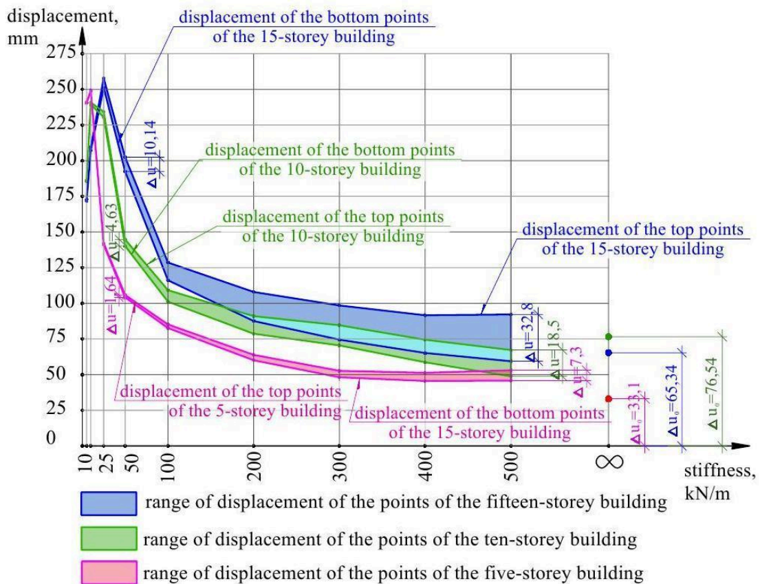
Фиг. 6. Обхват на изместване на точките на пет, десет и петнадесет етажни сгради
