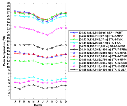
(kosong satu spasi tunggal, 12 pt) Gambar 1. Temperatur rata-rata bulanan AWS PTFI per ketinggian.
