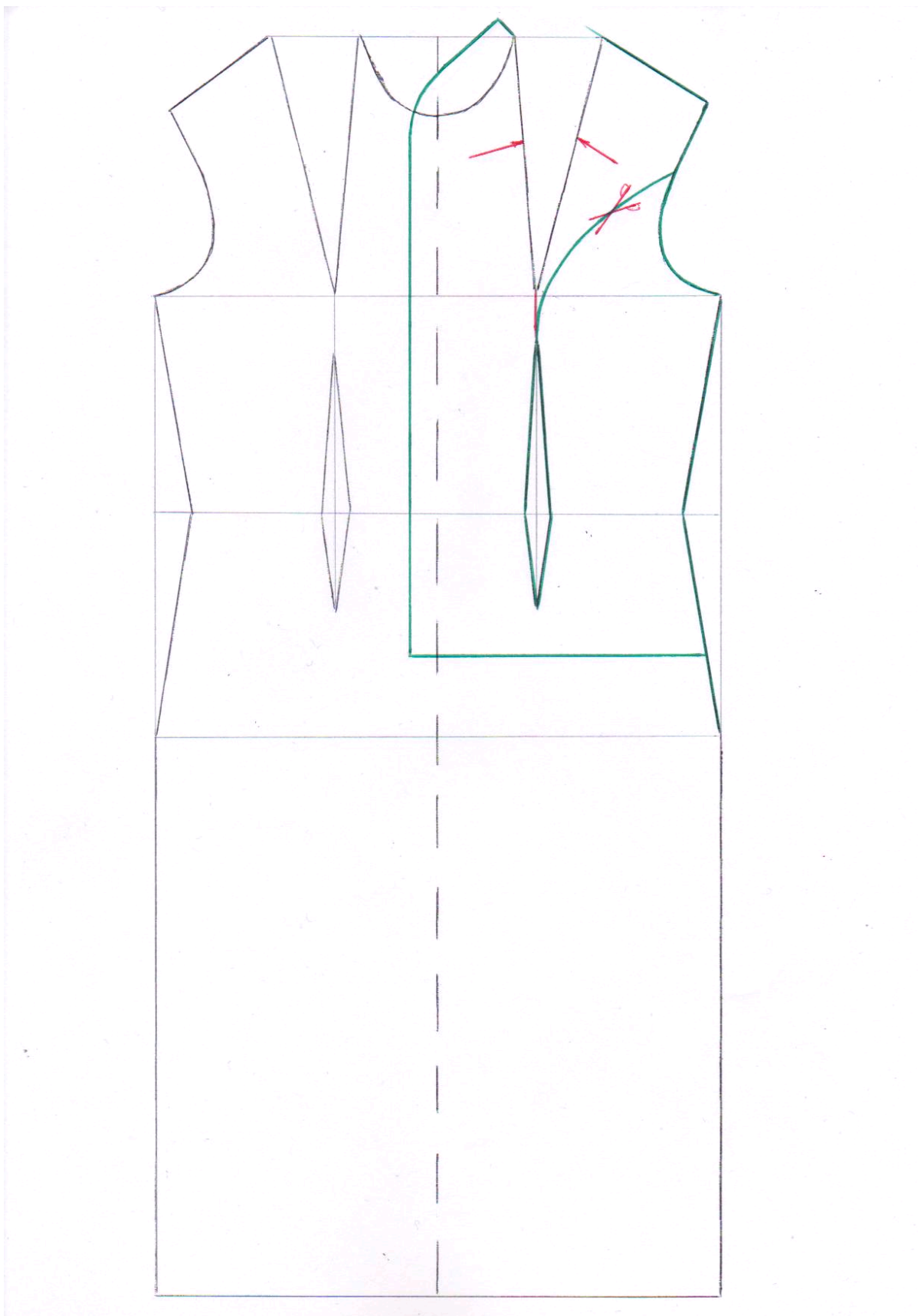
Рис. 39 Креслення лівої пілочки жакета моделі № 3
