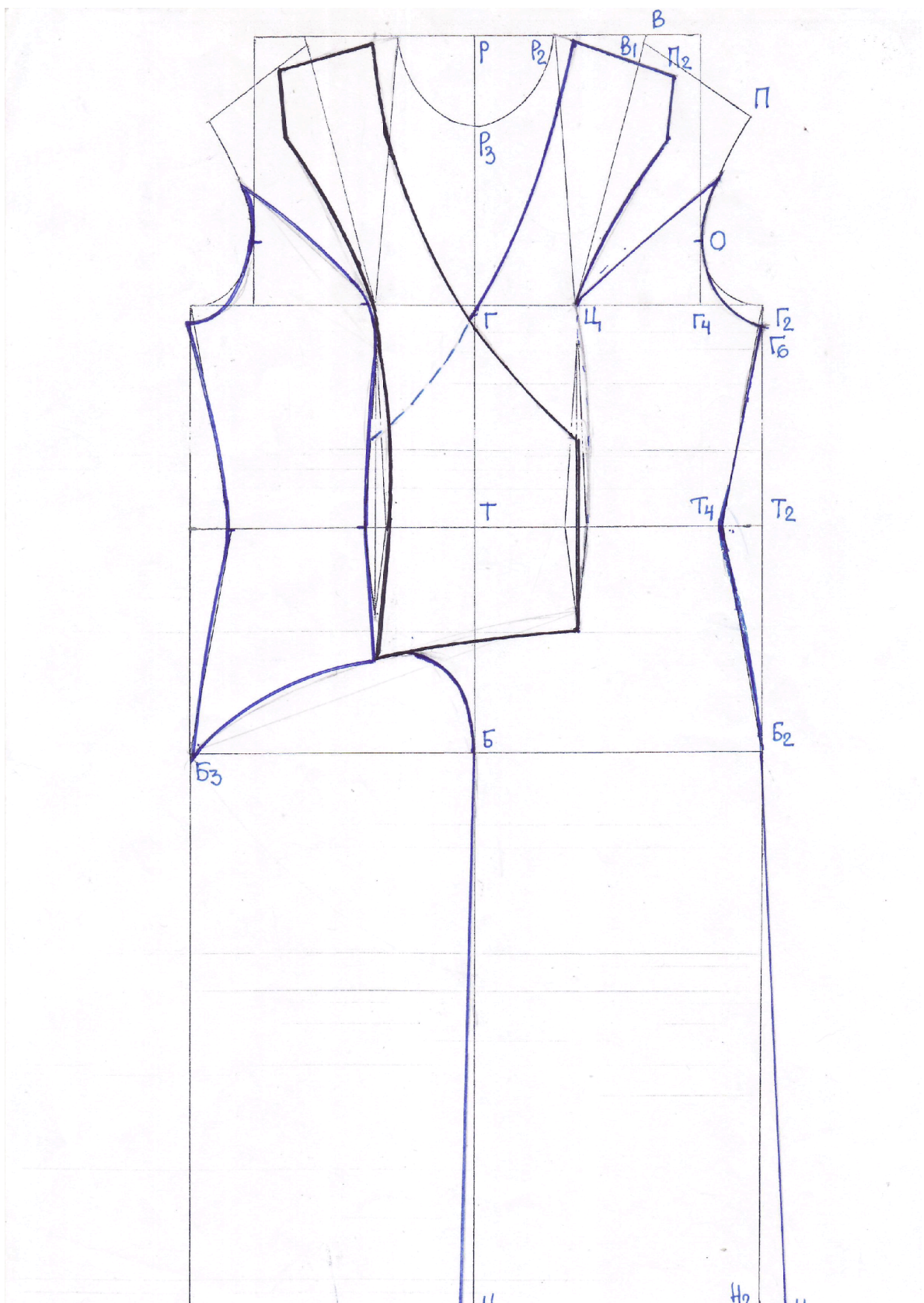
Рис.17 Креслення пілочки жилета моделі №1
