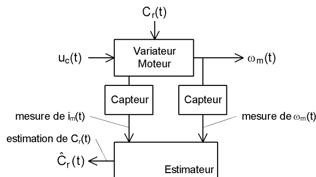
Fig. 10, architecture de la chaîne d'estimation
