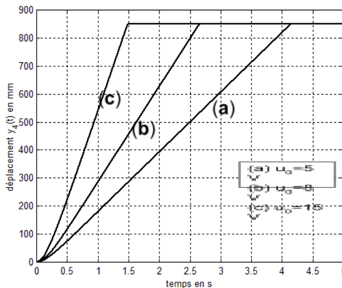
Fig. 7, réponse temporelle y_4(t)
