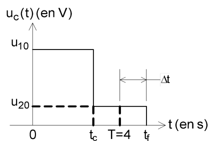
Fig. 8, définition du signal de commande u_c(t)
