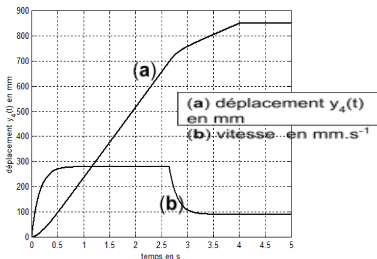
Fig. 9, évolution temporelle de y_4(t) et de \dot{y}_4(t)
