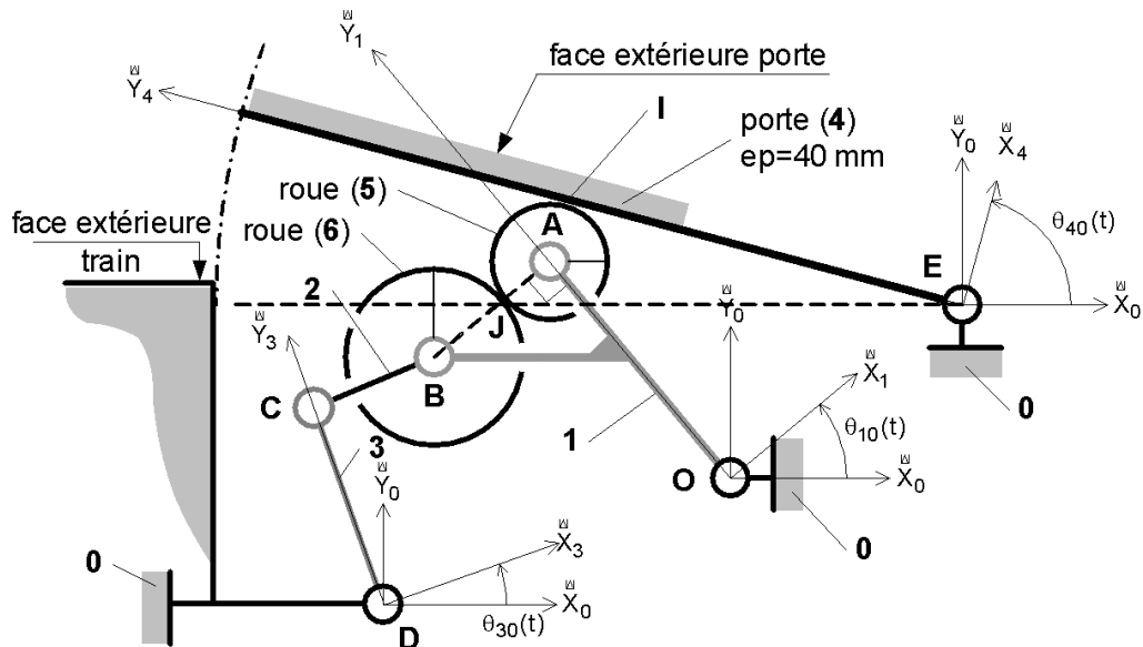
Fig. 4, schéma cinématique plan 'phase décalage en cours'
