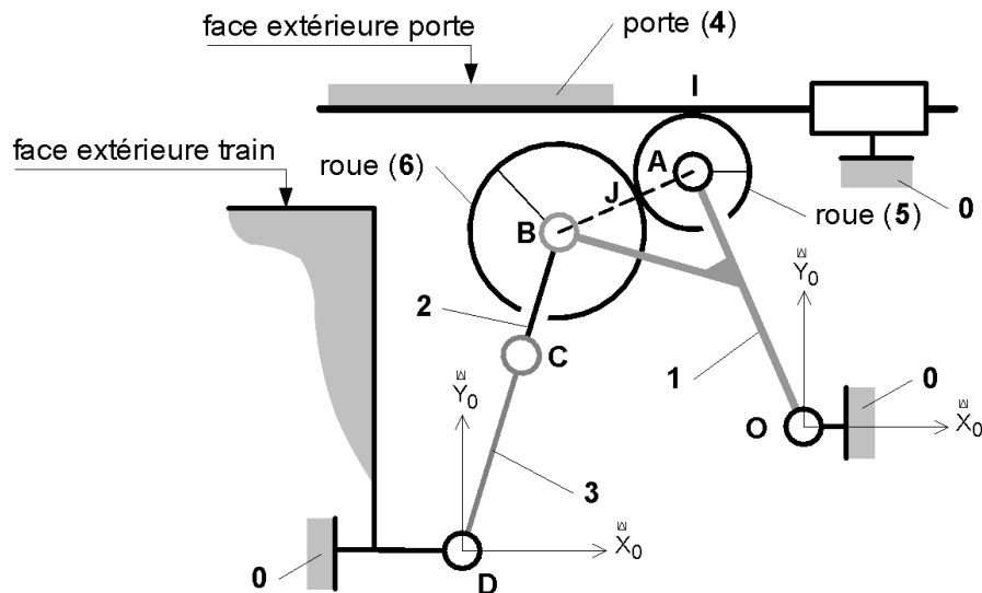
Fig. 5, schéma cinématique plan 'phase escamotage'
