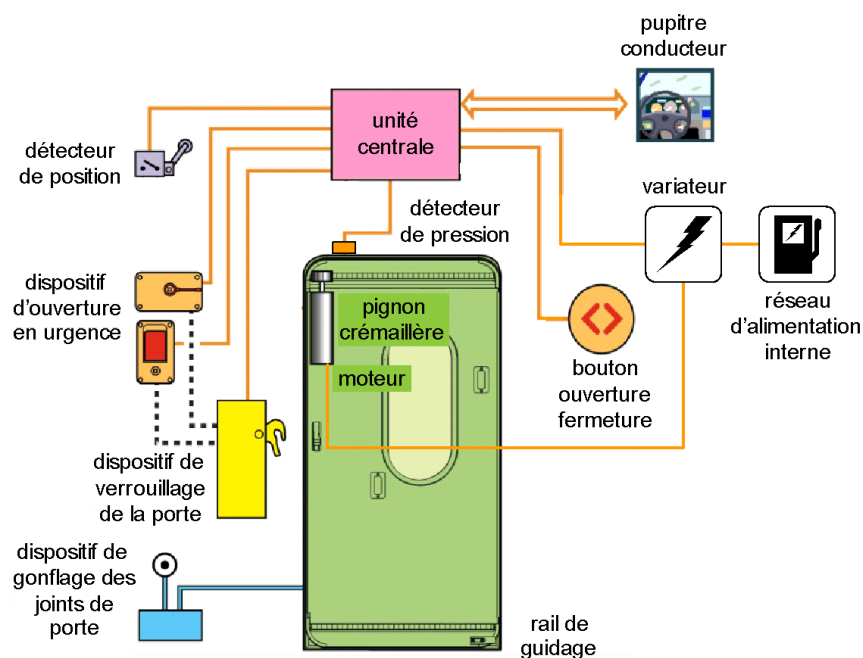
Fig. 1, interface fonctionnelle du système porte
