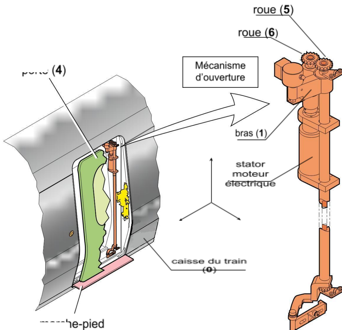
Fig. 2, architecture générale
