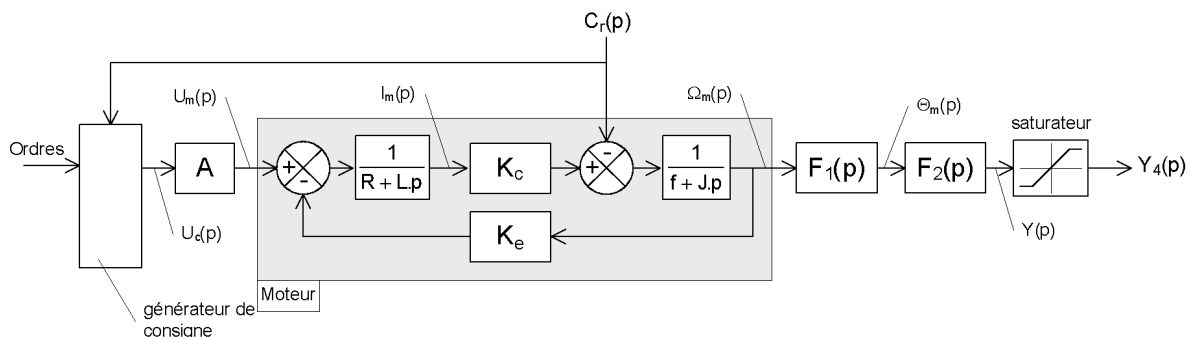
Fig. 6, modèle de commande
