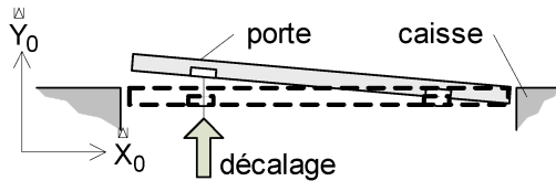
Fig. 3a, phase de décalage
