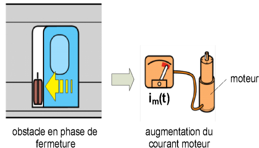
Fig. 13, principe de protection en phase de fermeture
