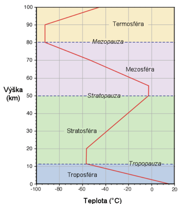
vrstvy atmosféry
