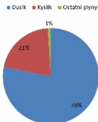
zloženie vzduchu
