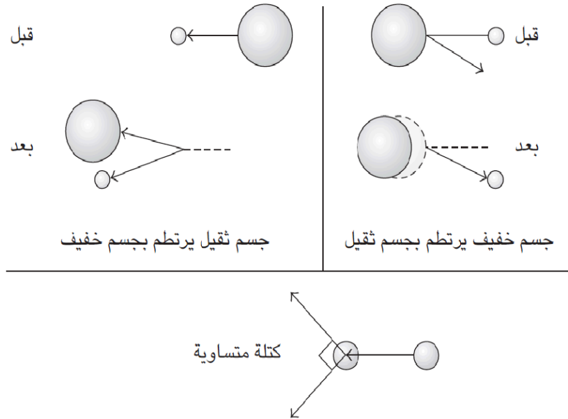
شكل ٣-١: نتائج ارتطام الأجسام الثقيلة والخفيفة بالأجسام الخفيفة والثقيلة، على الترتيب.
