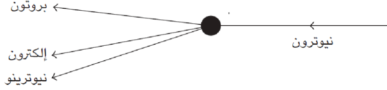
شكل ٤-٢: تحلل بيتا للنيوترون.
