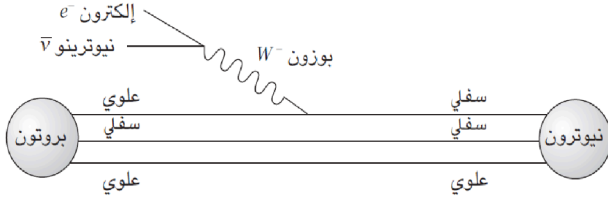
شكل ٧-٢: تحلل بيتا عن طريق البوزون W^- : يتحول النيوترون إلى بروتون عن طريق إطلاق بوزون W^- ، الذي يتحول بعد ذلك إلى إلكترون ونيوترينو.
