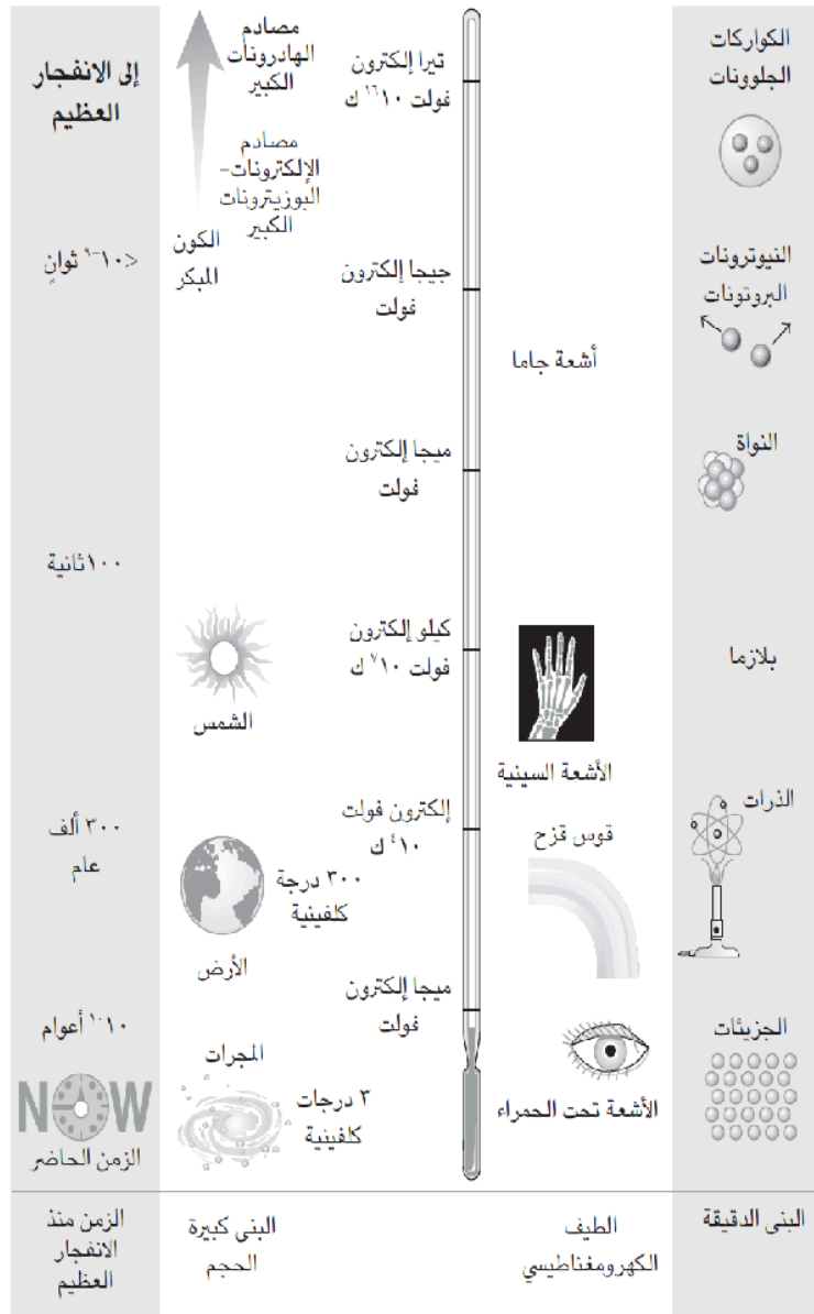
شكل ٢-٢: التوافق بين مستويات درجات الحرارة والطاقة بالإلكترون فولت.
