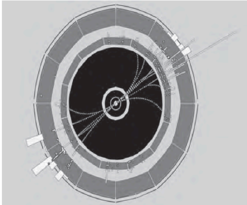
شكل ٦-٦: آثار من الجسيمات والجسيمات المضادة كما تظهر على شاشة الكمبيوتر. قارن الصورة على شاشة الكمبيوتر بالصورة الفعلية للكاشف في الشكل ٦-٥.
