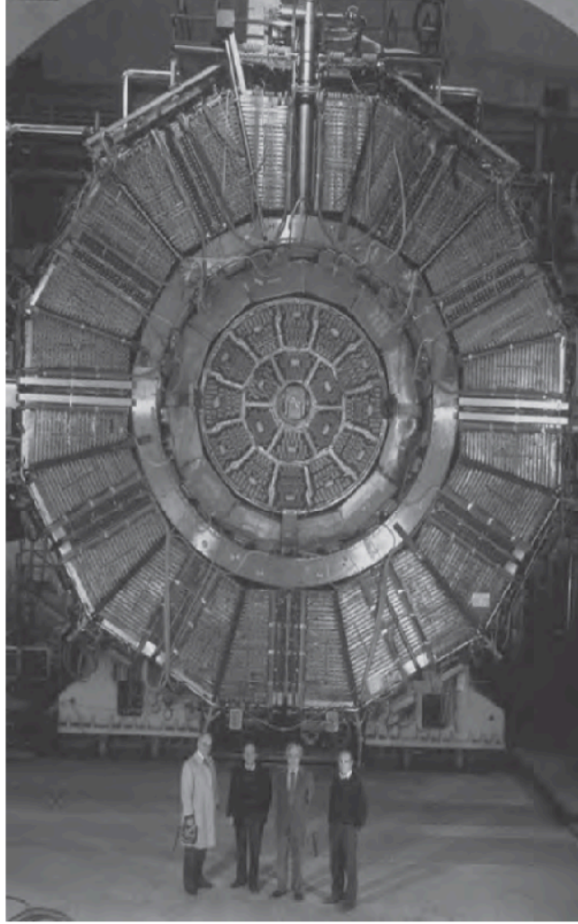
شكل ٥-٦: أحد الكواشف في مصادم الإلكترونات-البوزيترونات الكبير وإلى جواره أربعة من العلماء، ويتضح من الصورة حجم الكاشف. 4
