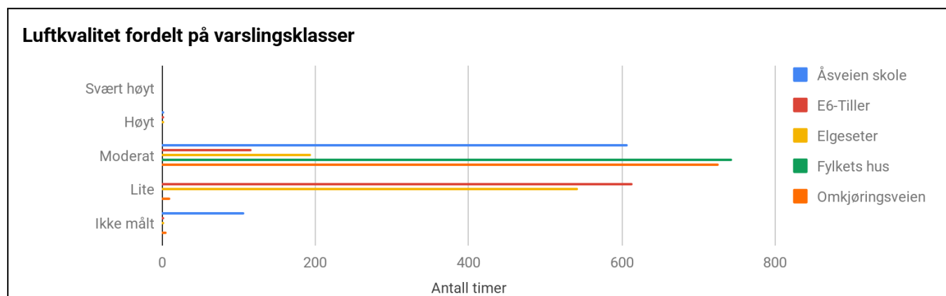
Figur 1 gir en totalvurdering av luftkvaliteten basert på alle timeverdier for svevestøv ( PM_{10} og PM_{2,5} ) og nitrogen-dioksidd ( NO_2 ), jf. varslingsklassene. Se også figur 2, 3 og 5. NB: “Moderat” forurensningsnivå er ikke alltid reelt 1
